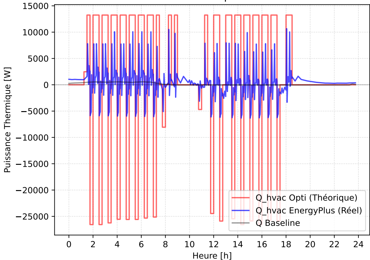
Courbes Flux Thermique - 2025-10-04
