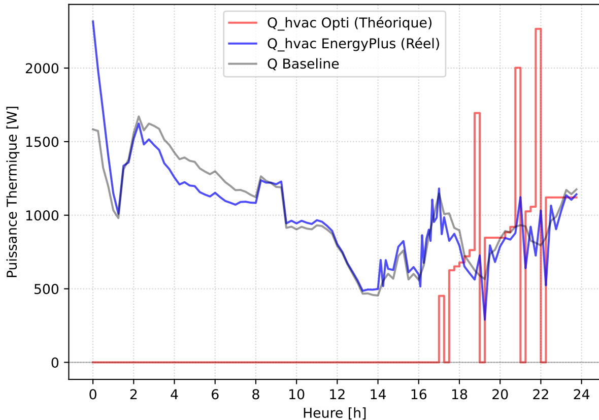
Courbes Flux Thermique - 2025-11-22
