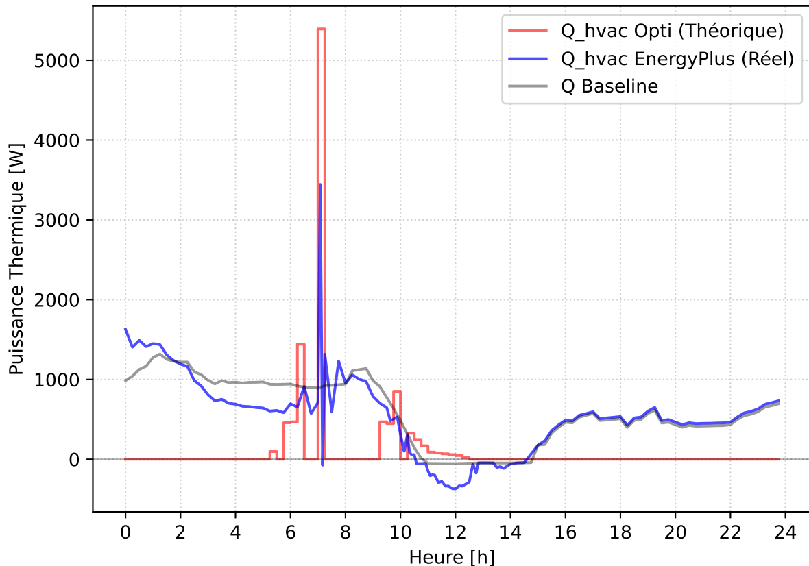
Courbes Flux Thermique - 2025-12-24
