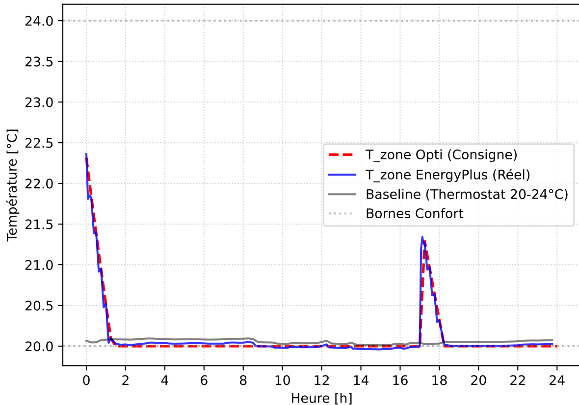
Courbes Températures - 2025-02-04
