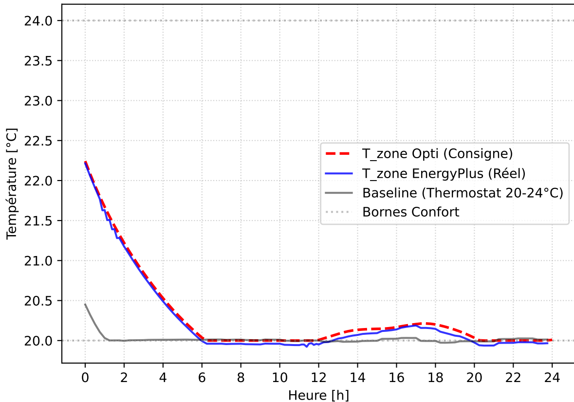
Courbes Températures - 2025-03-01
