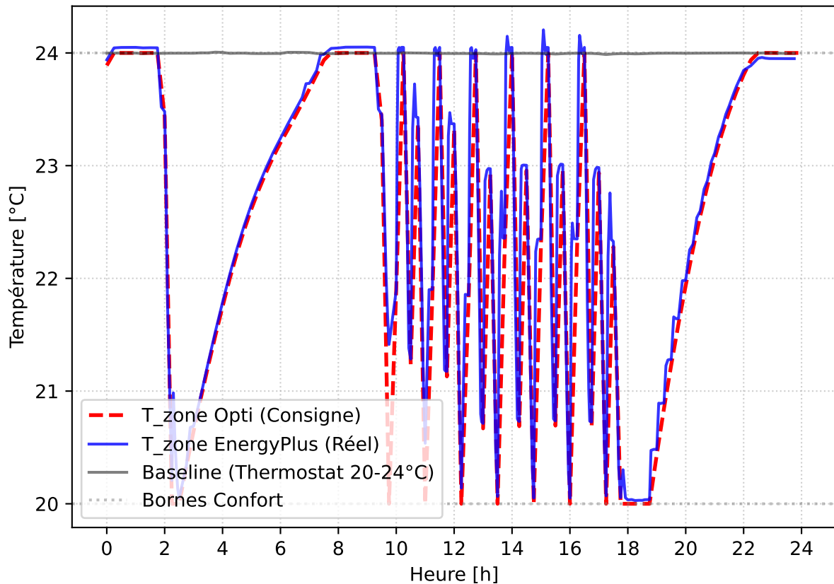
Courbes Températures - 2025-08-05
