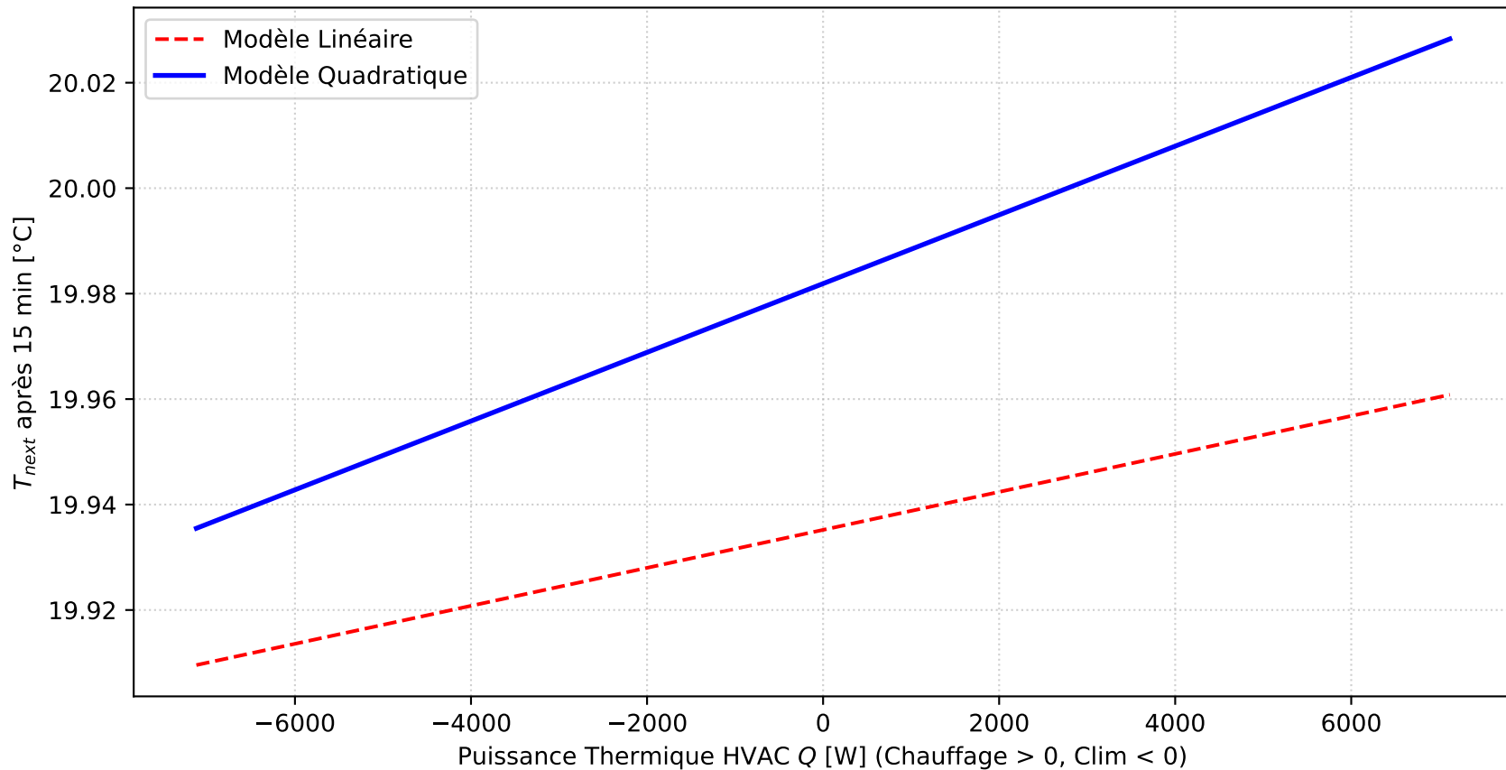
Coupe Thermique : Impact de Qhvac (Q) à T_{in}=20.0^{\circ}\text{C} et T_{out}=-5.0^{\circ}\text{C}
