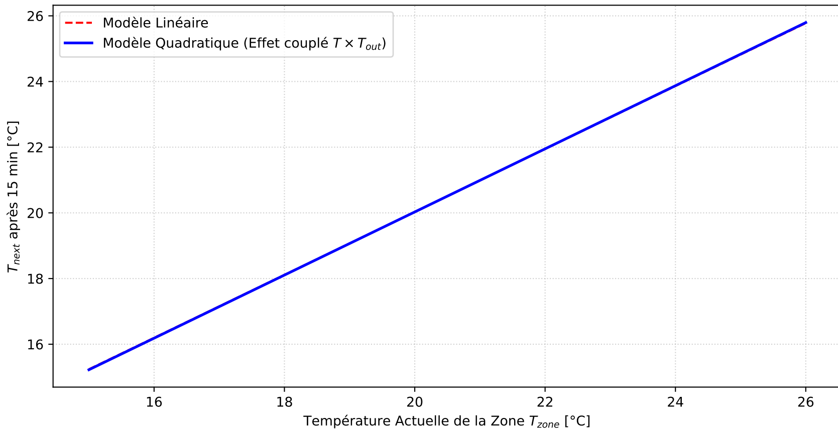
Coupe Thermique : Sensibilité à T_{zone} ( Q=3000.0W , T_{out}=5.0^{\circ}C )
