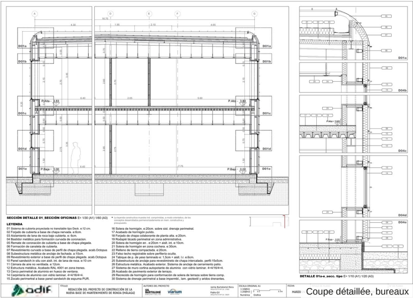
Coupe détaillée, bureaux
