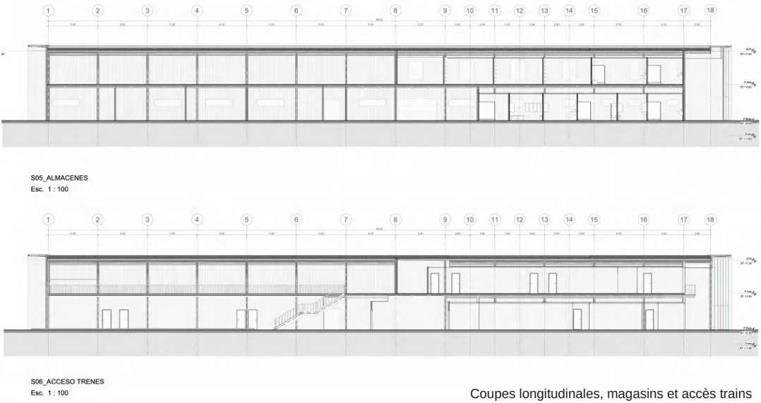
Coupes longitudinales, magasins et accès trains
