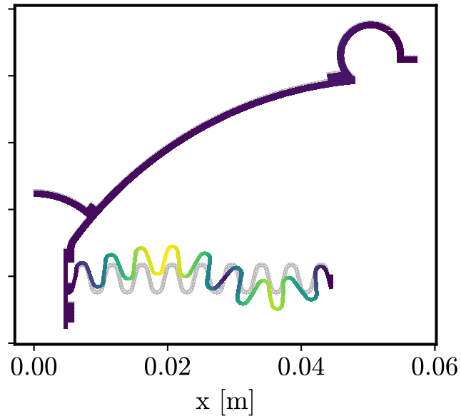
Mode 3 419.2 Hz \zeta=0.0432
