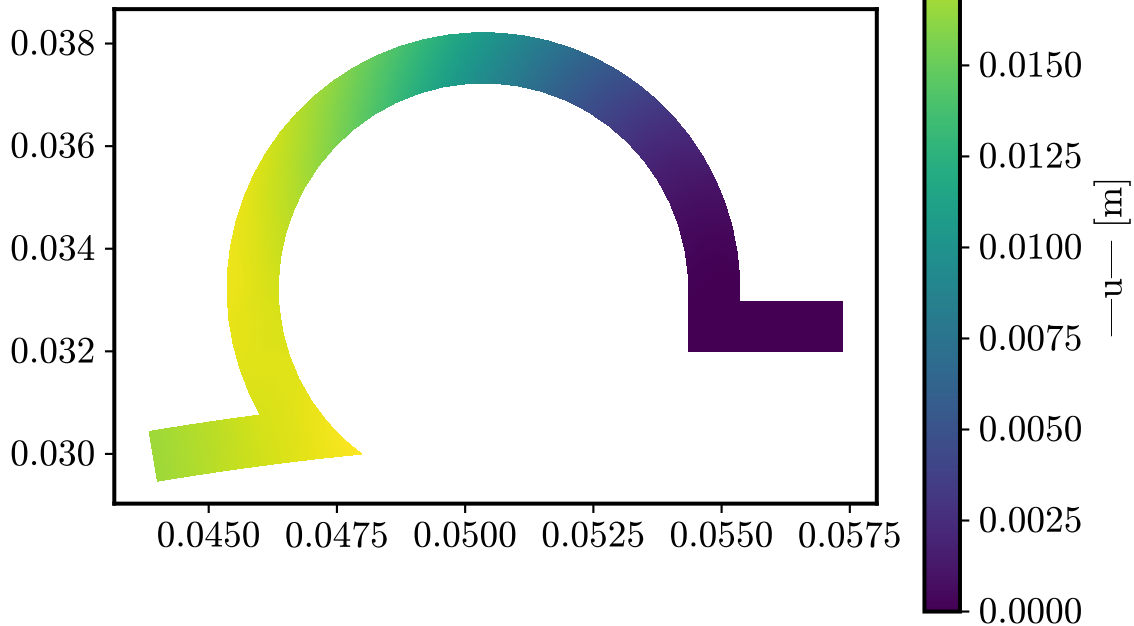
Cone - mode 3 - 419.2 Hz
