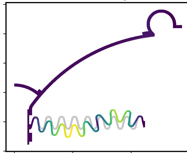
Mode 3 419.2 Hz \zeta=0.00873
