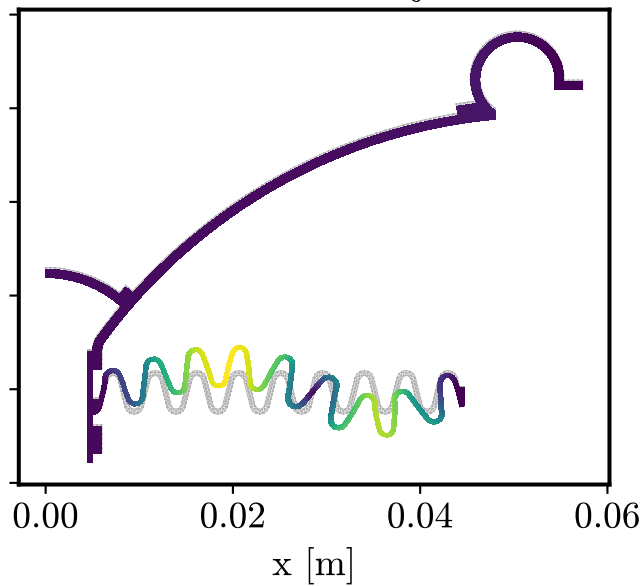
Mode 3 419.2 Hz \zeta=0.0432
