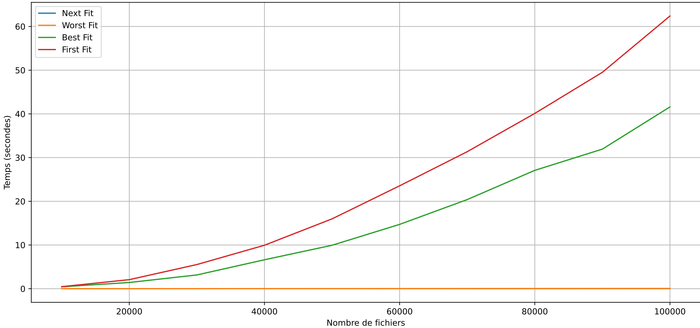
Comparaison du temps de calcul
