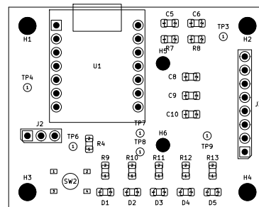
VIBRA Rev E-HS / Assemblage - vue de dessus
