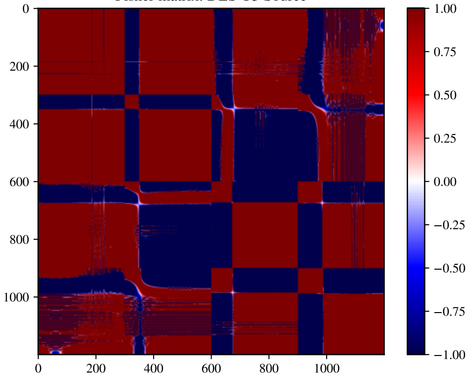
Fisher matrix: DES Y3 Source
