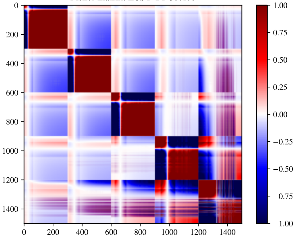
Fisher matrix: LSST Y1 Source
