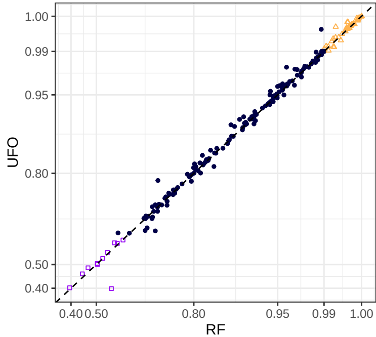
AUC
