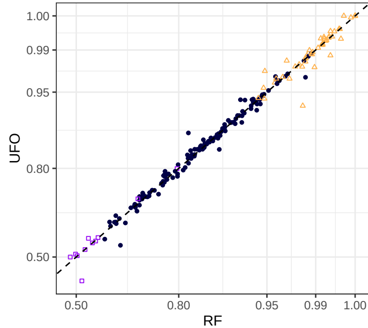
ACC
