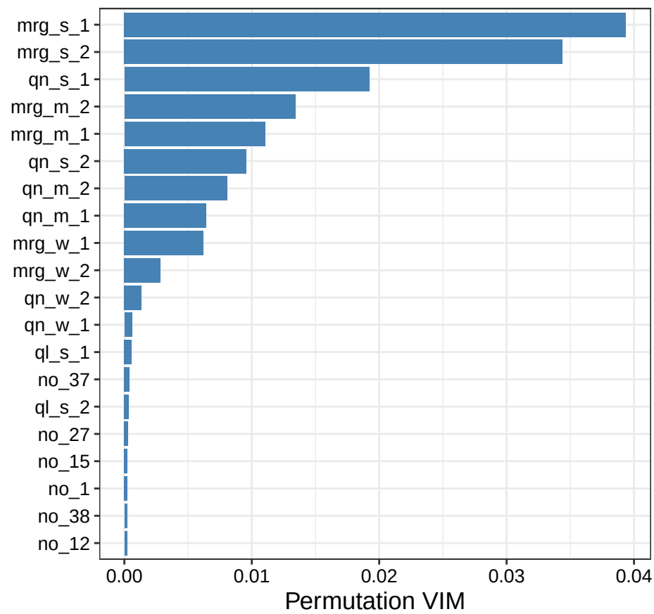
DGP 2
