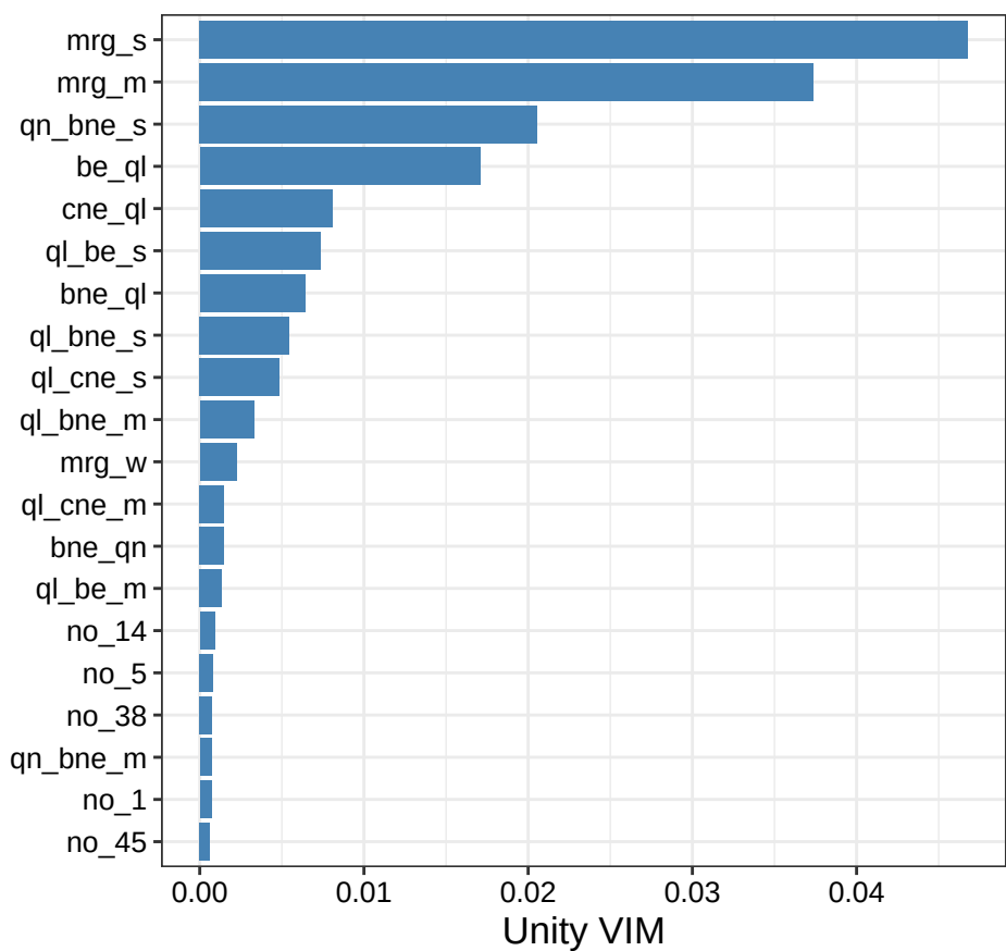
DGP 2
