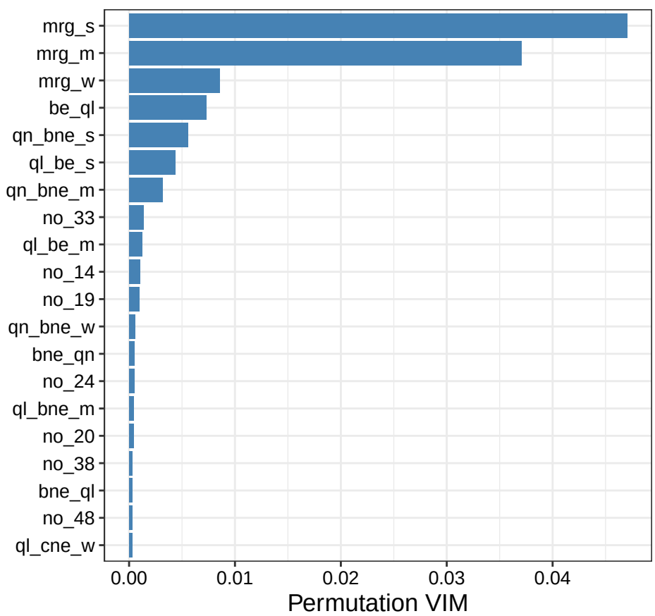
DGP 2
