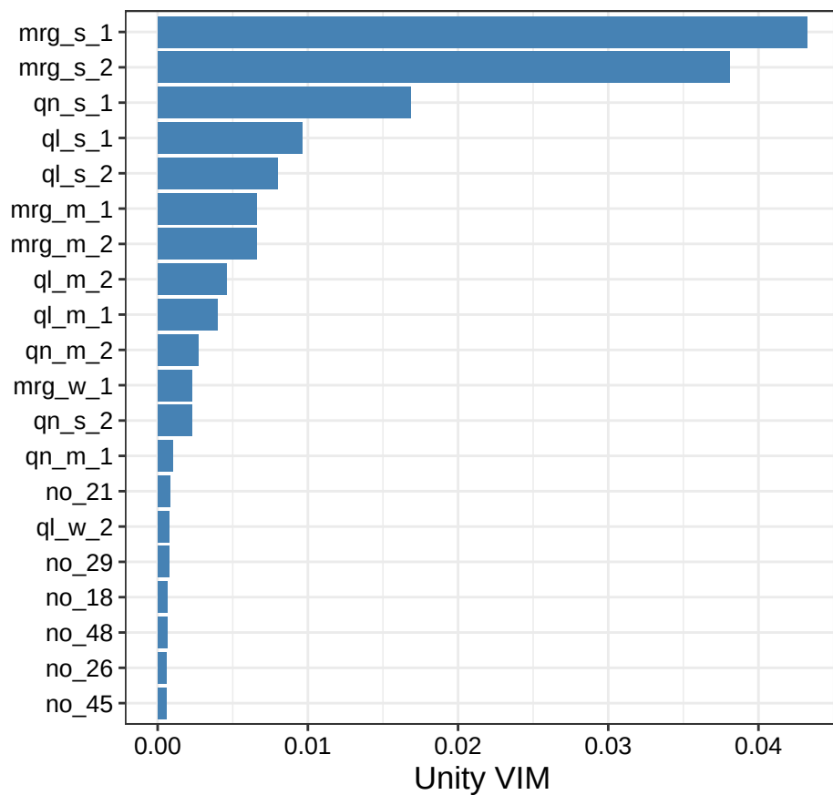
DGP 2
