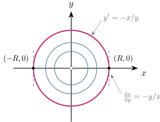
Рис. 1.13: Окружности x^2 + y^2 = R^2 — интегральные кривые формы F = x dx + y dy в G = \mathbb{R}^2 \setminus \{(0, 0)\} . Там, где y \neq 0 , форма равносильна уравнению y' = -x/y , а в двух точках (\pm R, 0) касательная вертикальна (пунктир) и вместо него работает \frac{dx}{dy} = -y/x . Условие m^2 + n^2 \neq 0 гарантирует, что в каждой точке применимо хотя бы одно из них, — поэтому симметричная форма описывает окружность целиком, а не по половине.
