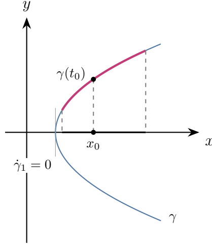
Рис. 1.12: Участок кривой \gamma , на котором \dot{\gamma}_1 \neq 0 (выделен): там кривая однозначно проецируется на ось Ox и является графиком функции y(x) . В точке, где \dot{\gamma}_1 = 0 , касательная вертикальна и такой записи нет — поэтому переход к уравнению y' = -m/n возможен лишь локально.
