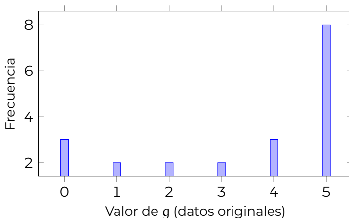
Figura 2: Distribución de los datos originales (no es normal).
