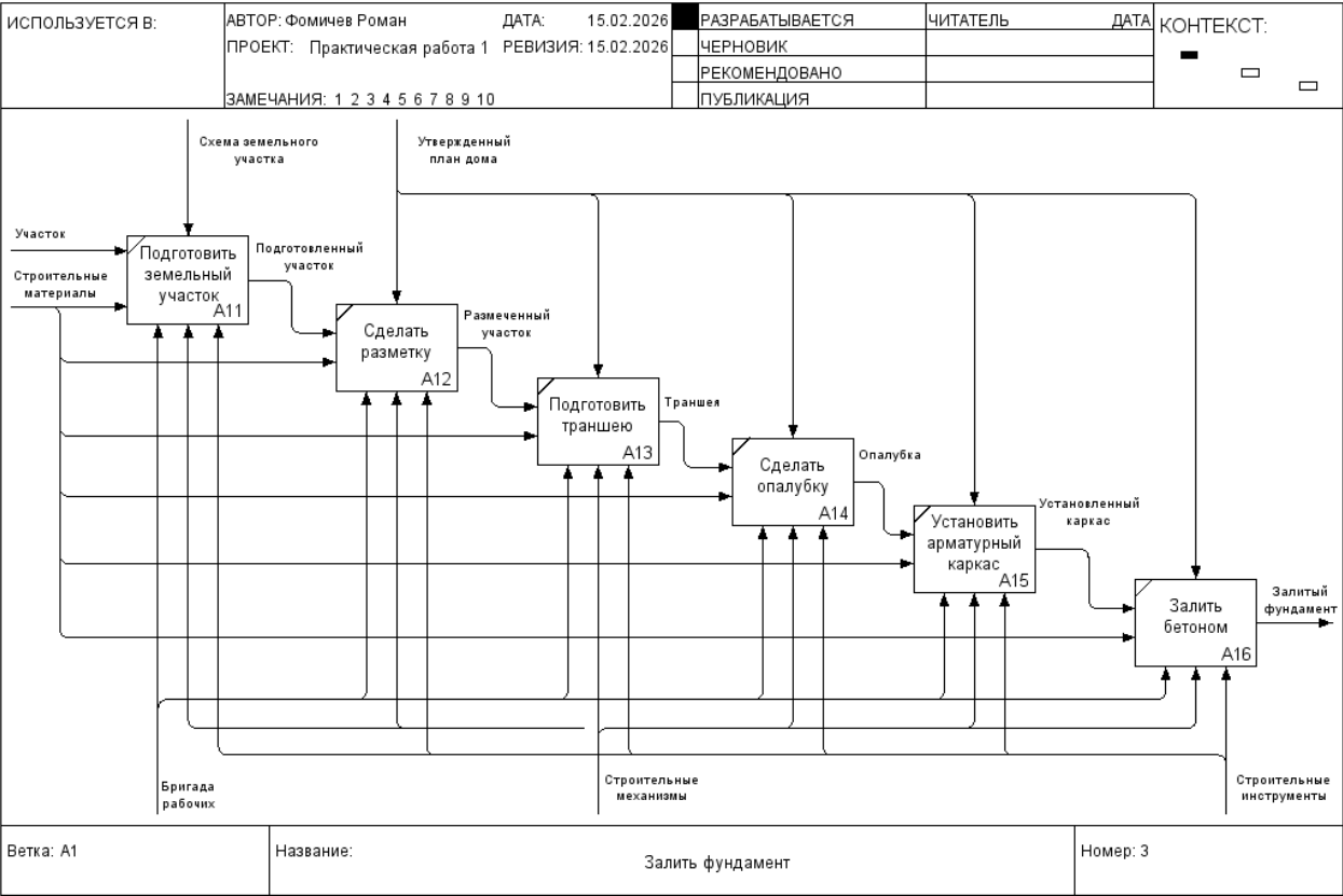
Рисунок 3 – Декомпозиция процесса «Залить фундамент»
