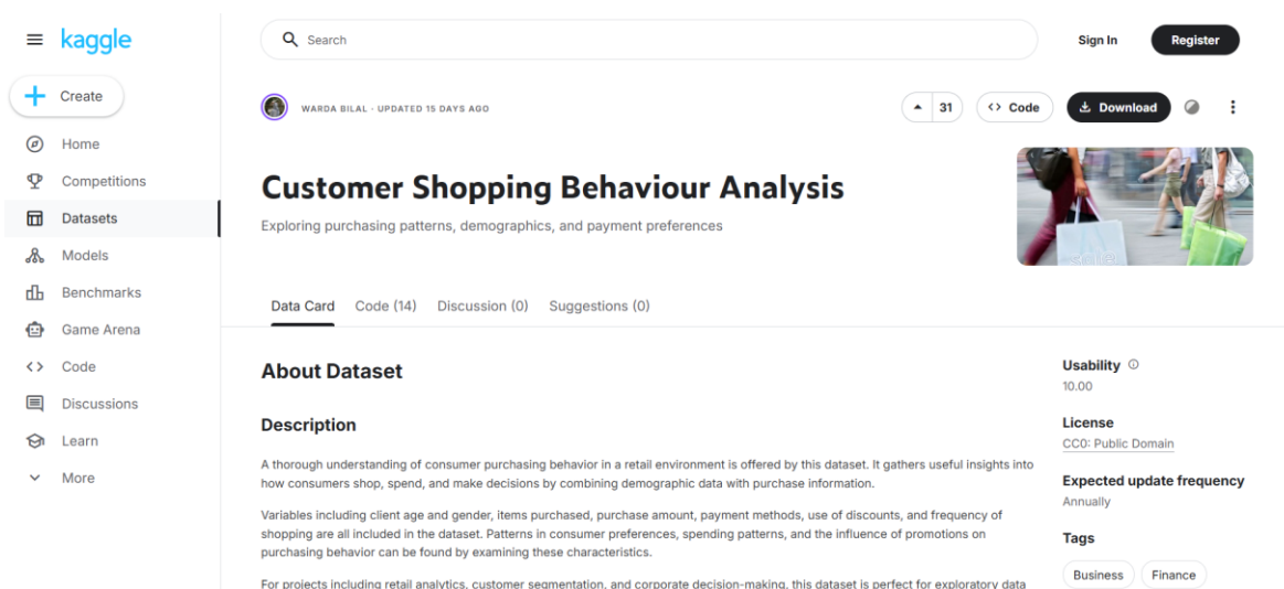
Рисунок 1 – Датасет
