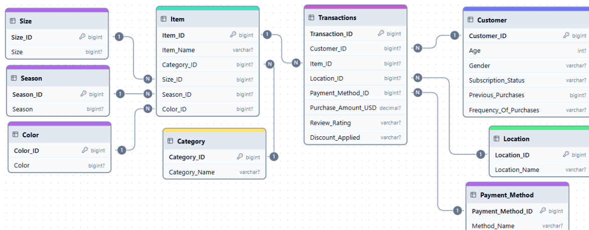
Рисунок 4 – Логическая модель в 5НФ
