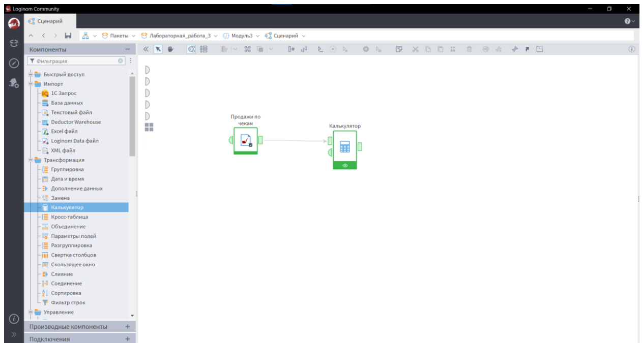
Рисунок 3 – Компонент “Калькулятор”
