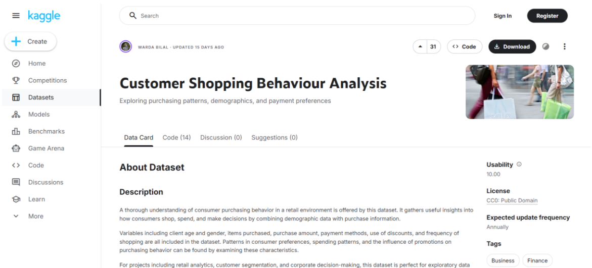
Рисунок 1 – Датасет
