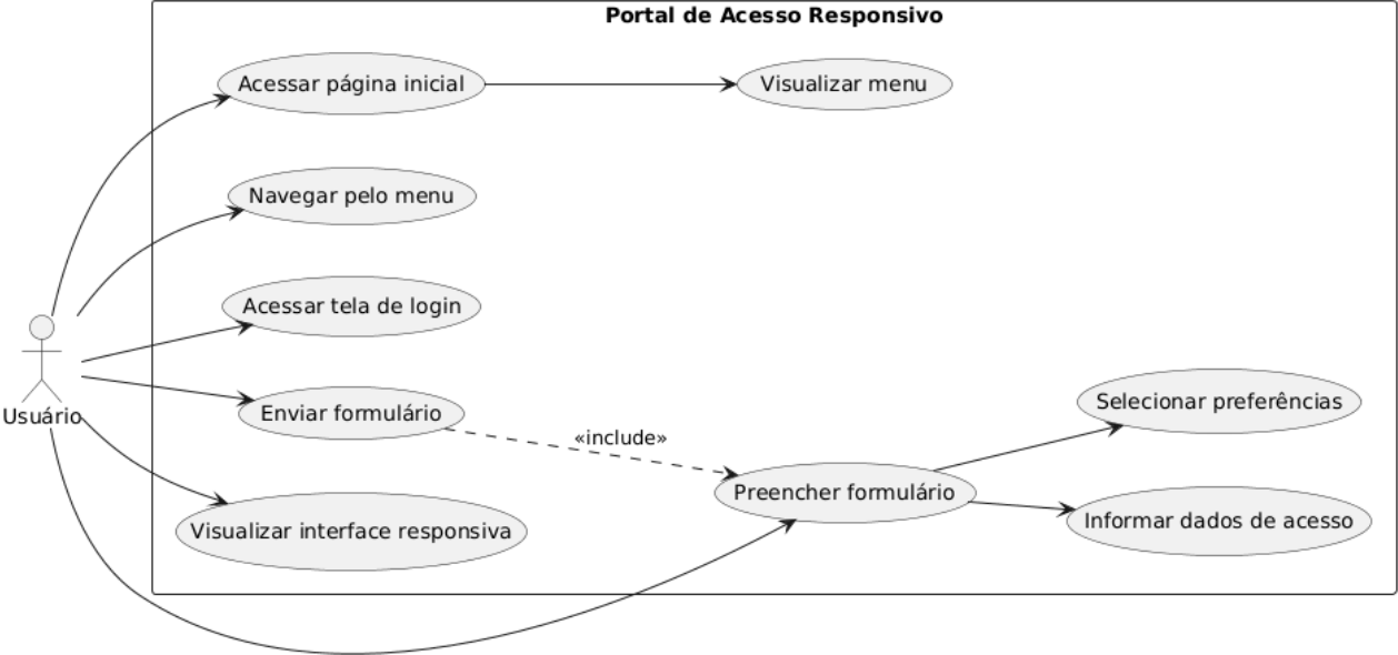
Diagrama de Casos de Uso - Portal de Acesso Responsivo
