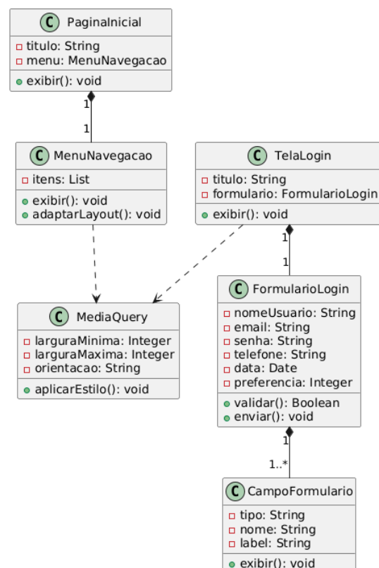
Diagrama de Classes - Portal de Acesso Responsivo
