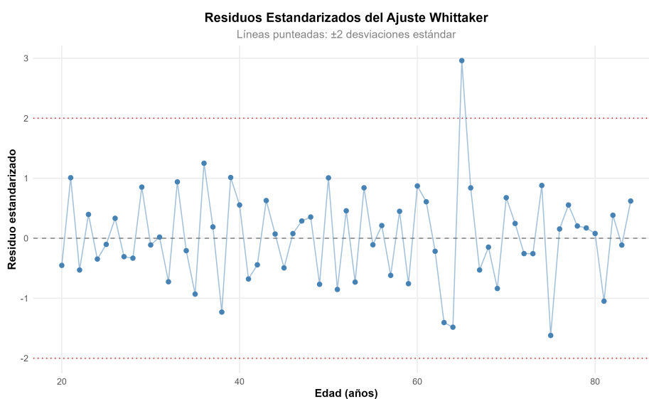
Figura 7: Residuos estandarizados del ajuste WH
