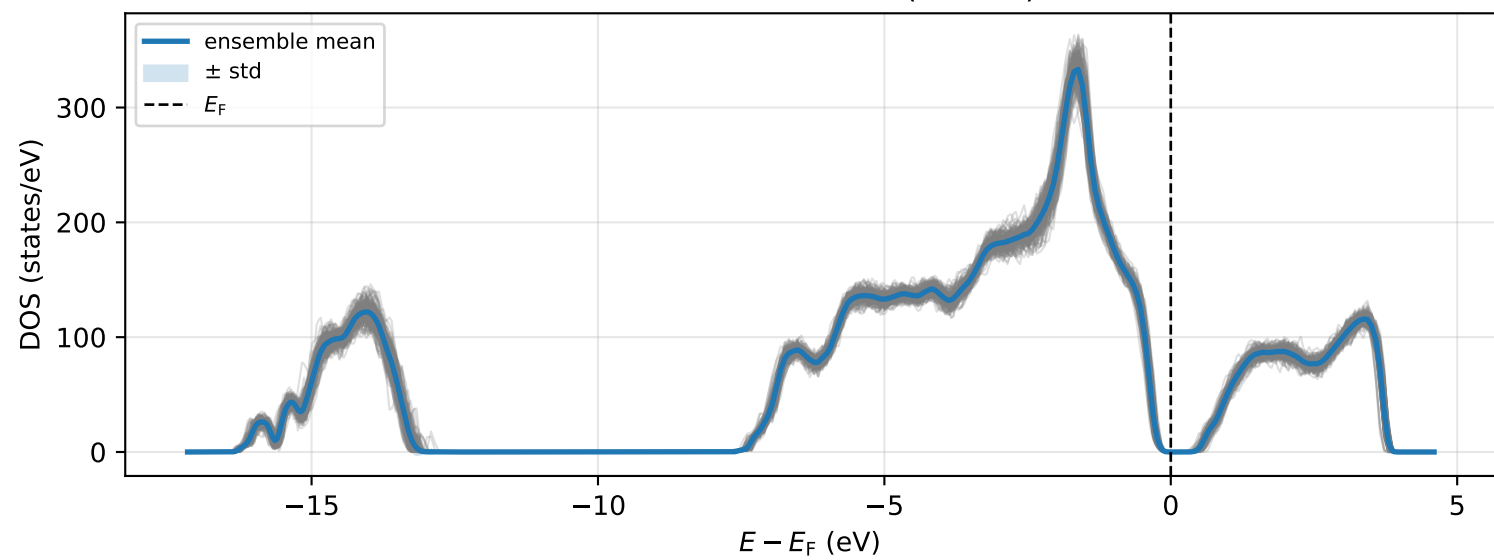
Total DOS — 650 K (n=150)
