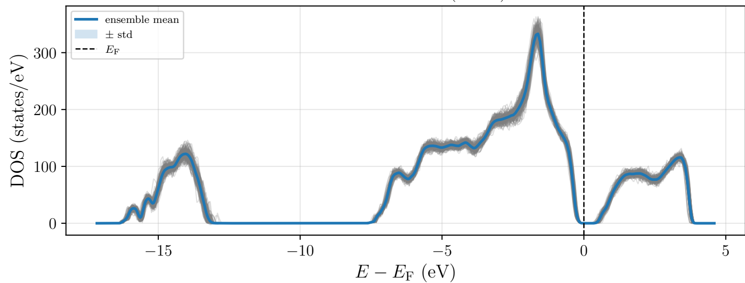
Total DOS — 650 K (n=150)
