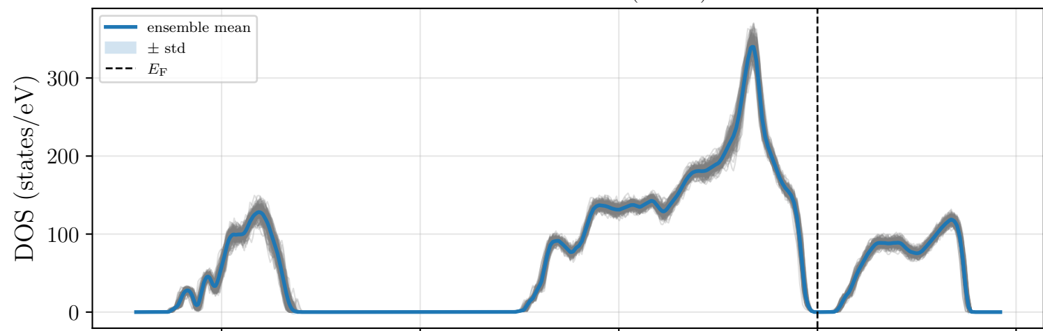
Total DOS — 650 K (n=150)
