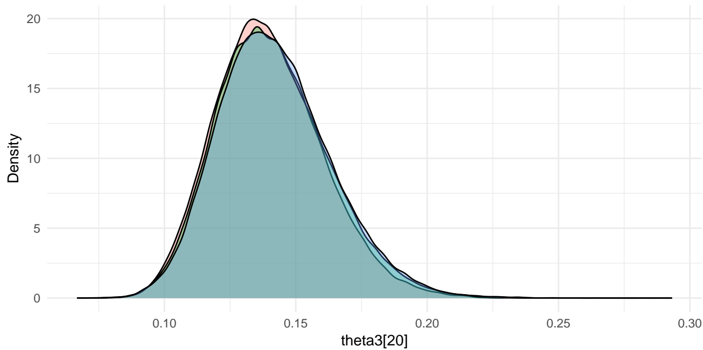
Density -- theta3[20]
