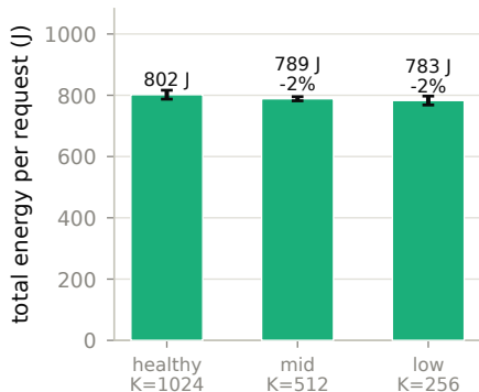
(d) CPU, 1024 output tokens: total energy
