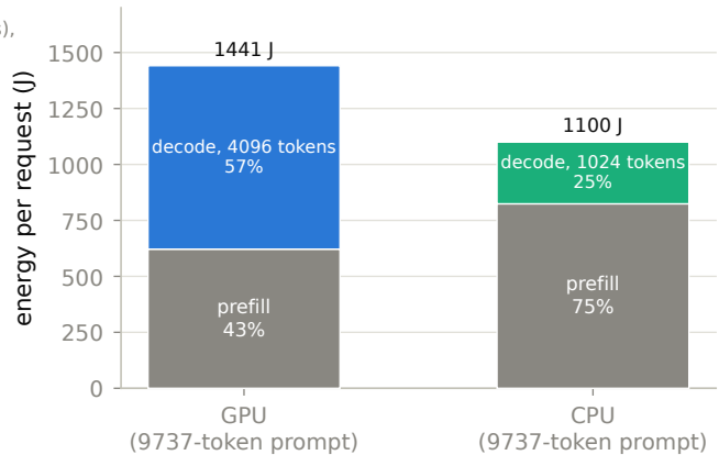
(d) where a request's energy goes
