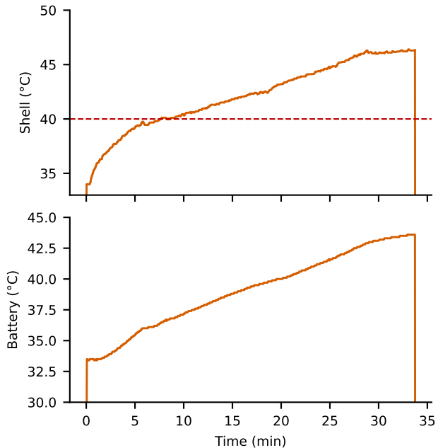
Bonsai-8B
