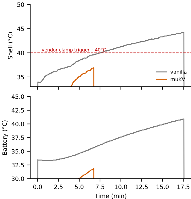
Llama-1B
