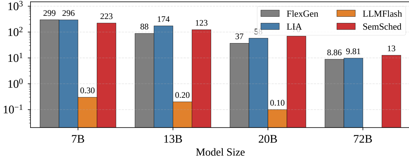
(b) Prefill Scalability, 32H+64C, (B=128)
