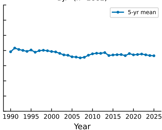
DJF (n=2882)
