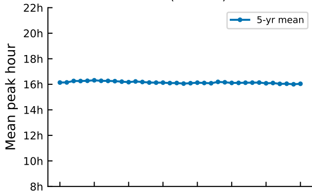
SON (n=3002)
