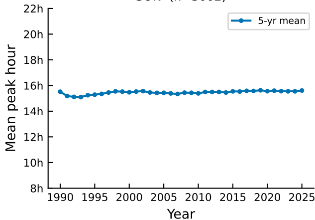
SON (n=3002)
