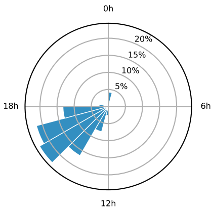
SON (n=3002)
