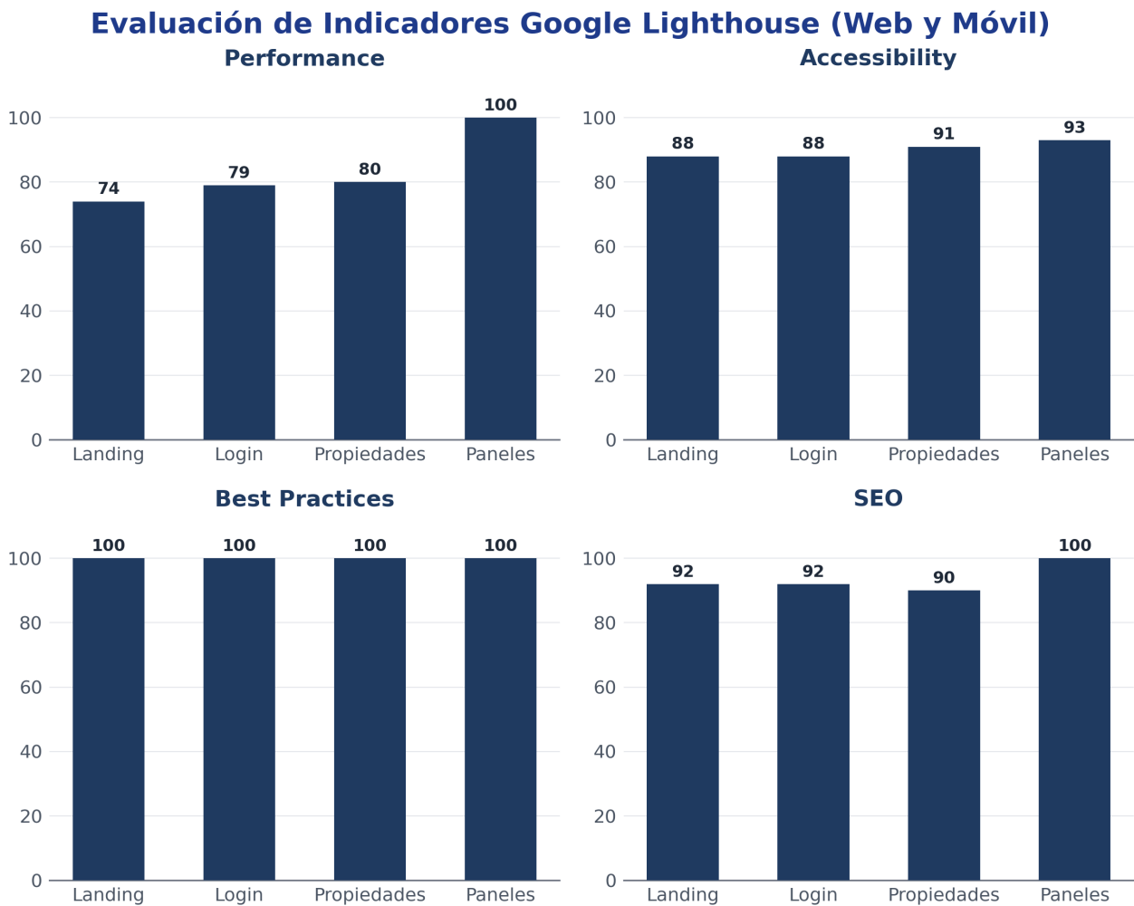
Figura 2: Calificación detallada de Google Lighthouse para cada dimensión evaluada por módulo.
