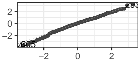
Normal Q-Q
