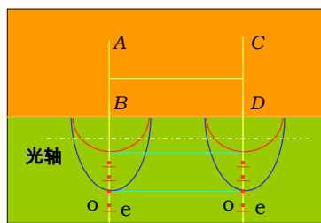
(d) 垂直入射, 光轴平行于晶面
