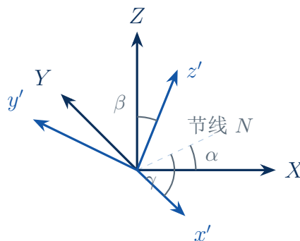
图 2: Euler 角 (zyz 约定) 的几何: 空间架 \{X, Y, Z\} 与本体架 \{x', y', z'\} 共原点, \alpha 是 X 轴与节线 N 的夹角 (进动), \beta 是 Z 轴与 z' 轴的夹角 (章动), \gamma 是节线与 x' 轴的夹角 (自转). 本体 z' 轴的方向完全由 (\alpha, \beta) 决定.
