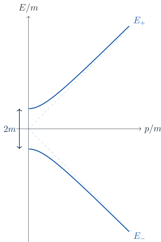
图 1: 自由 Dirac 粒子的色散关系(19.1): 正、负能量支与宽度 2m 的能隙; 虚线为光锥渐近线 E = \pm p (自然单位制下).
