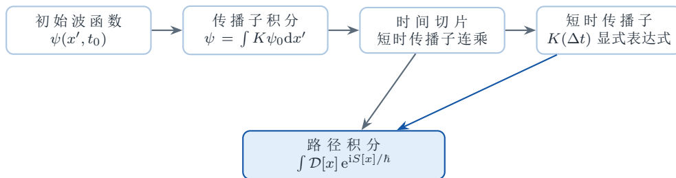
图 7: 第二章的推导链条. 从初始波函数出发, 经传播子积分得到任意时刻的波函数; 把传播子分解为短时传播子并求出其显式形式; 在连续极限下, 这些中间结果汇聚为路径积分(2.20).
