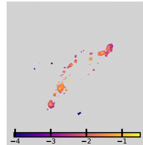
\log \Sigma_{\text{SFR}} (HII)
