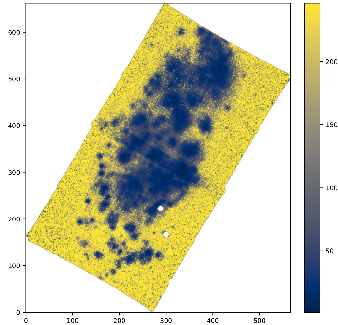
SPAXELS OIII5006_SIGMA_ERR
