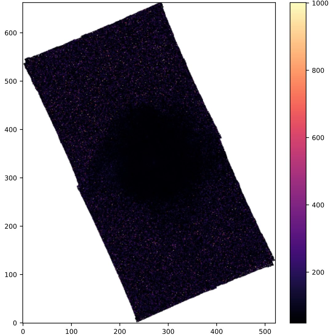
SPAXELS NII6583_SIGMA
