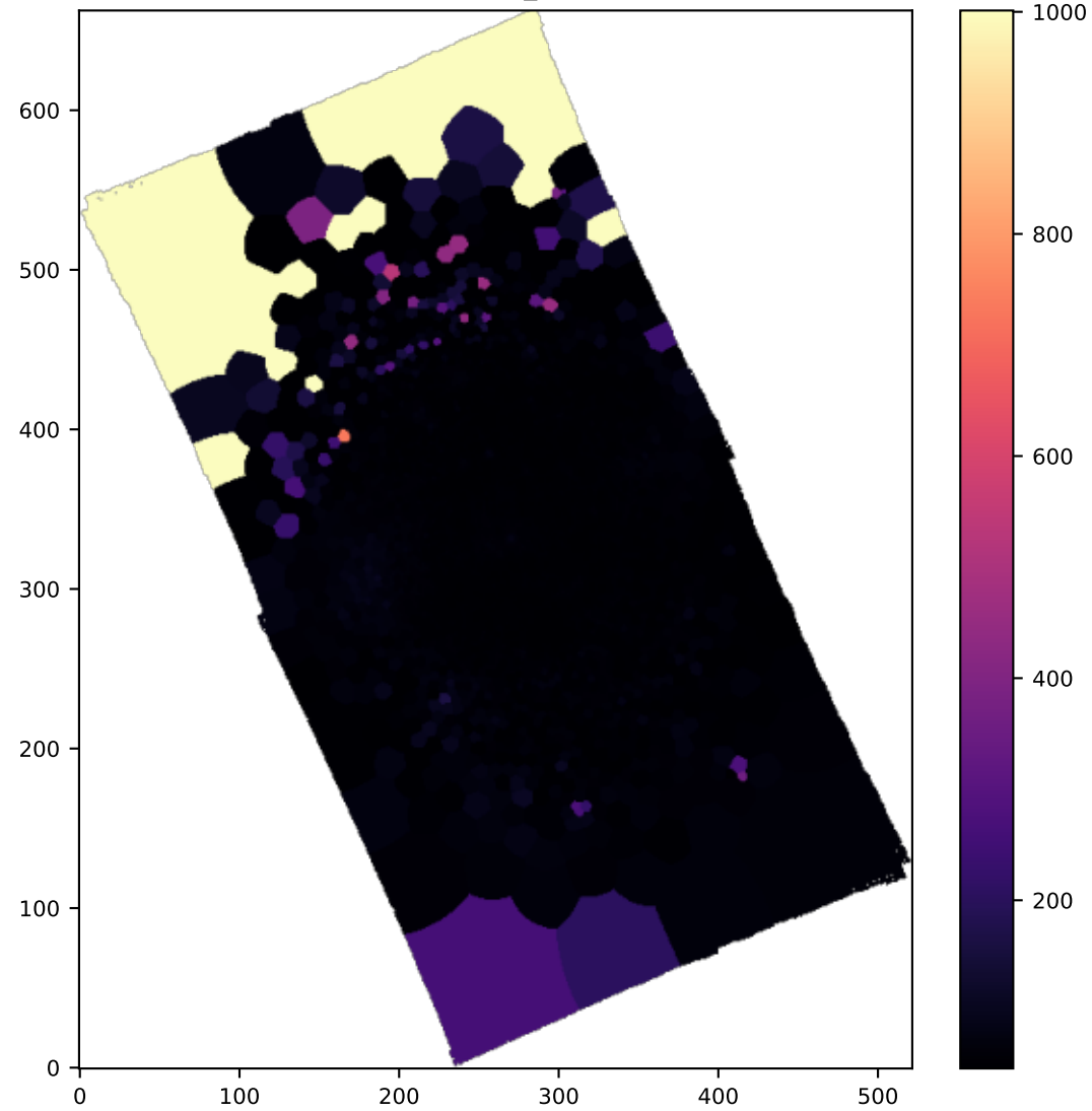
BIN NII6583_SIGMA
