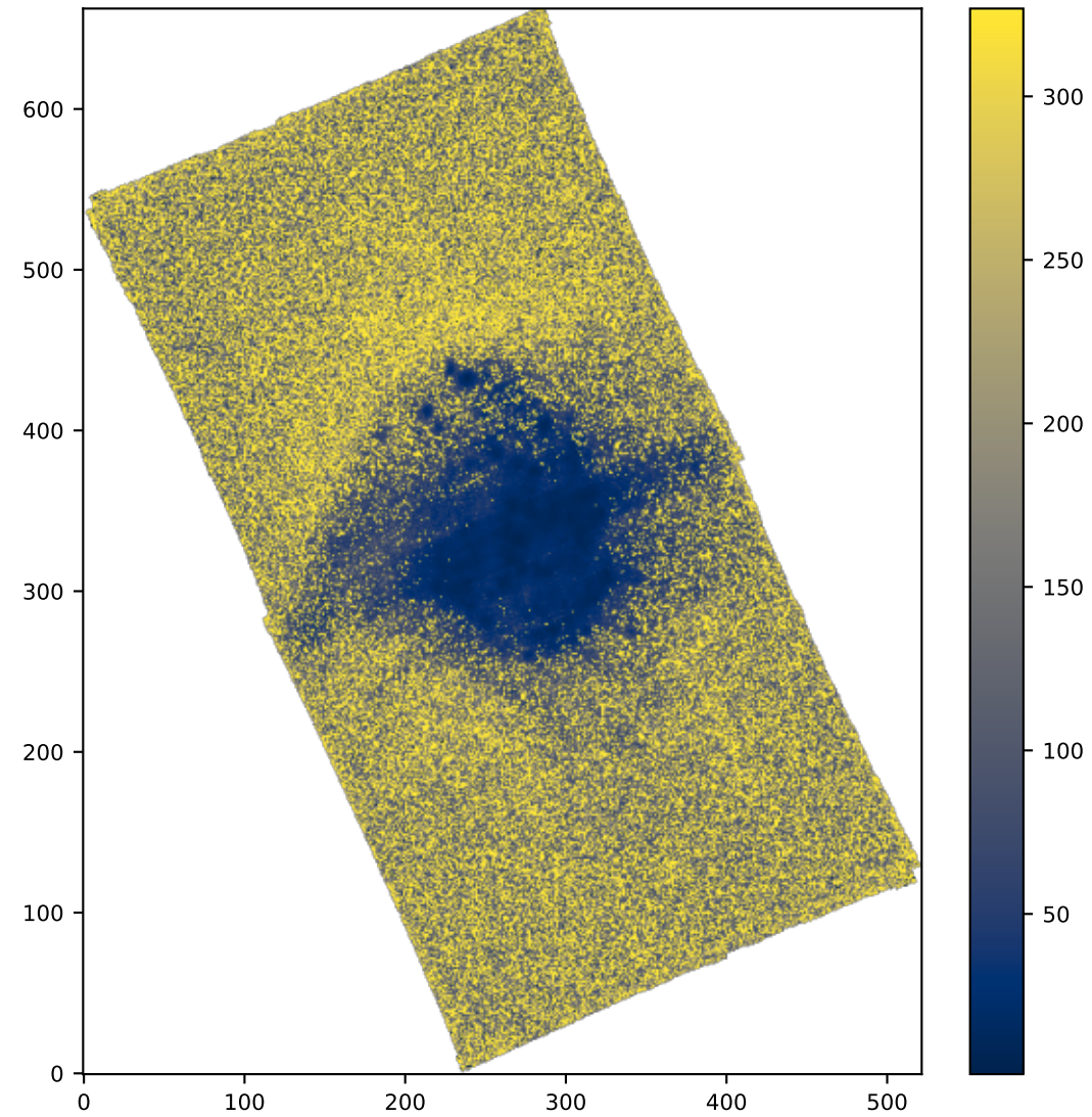
SPAXELS NII6583_SIGMA_ERR
