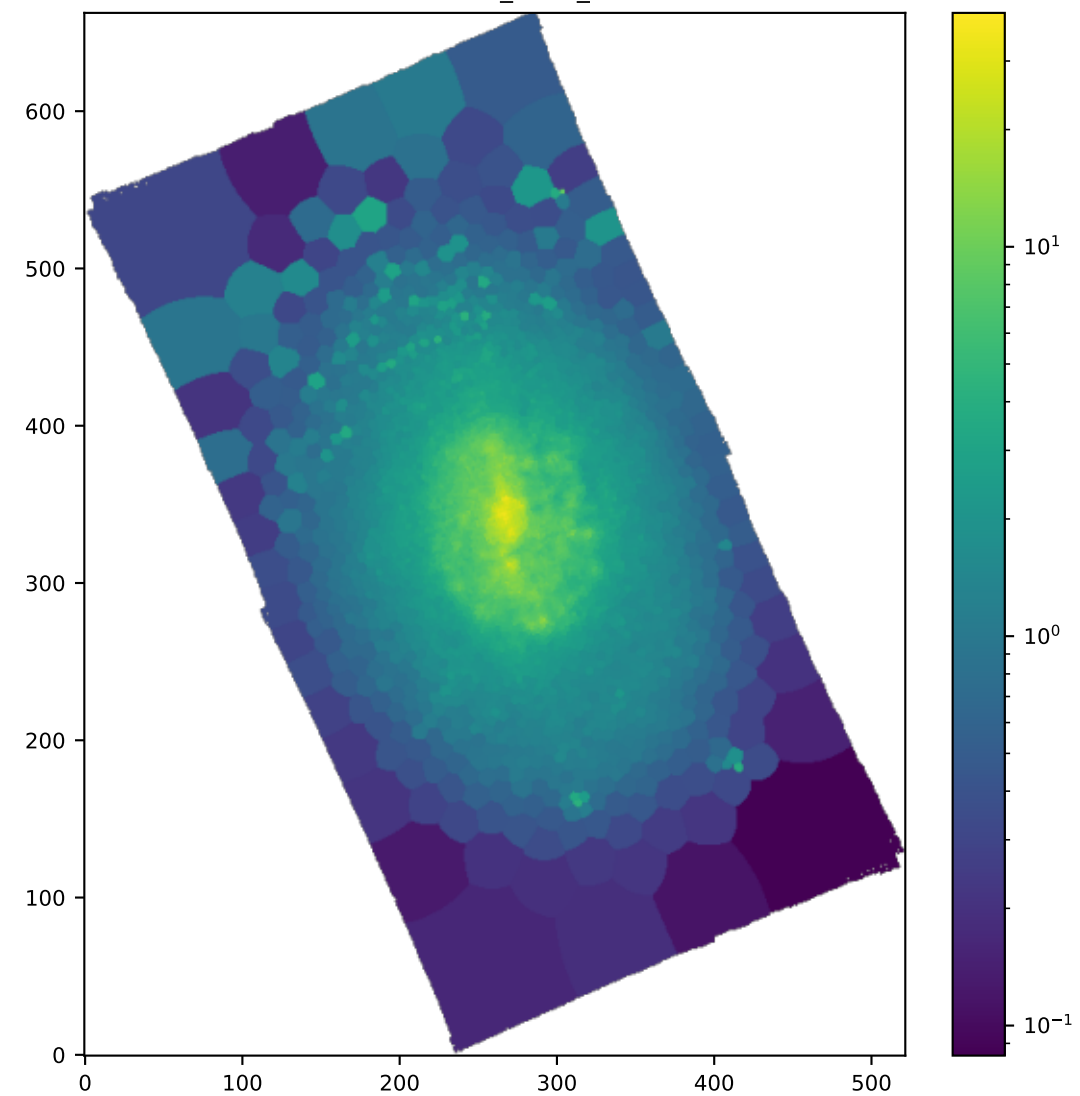
BIN NII6583_SIGMA_ERR
