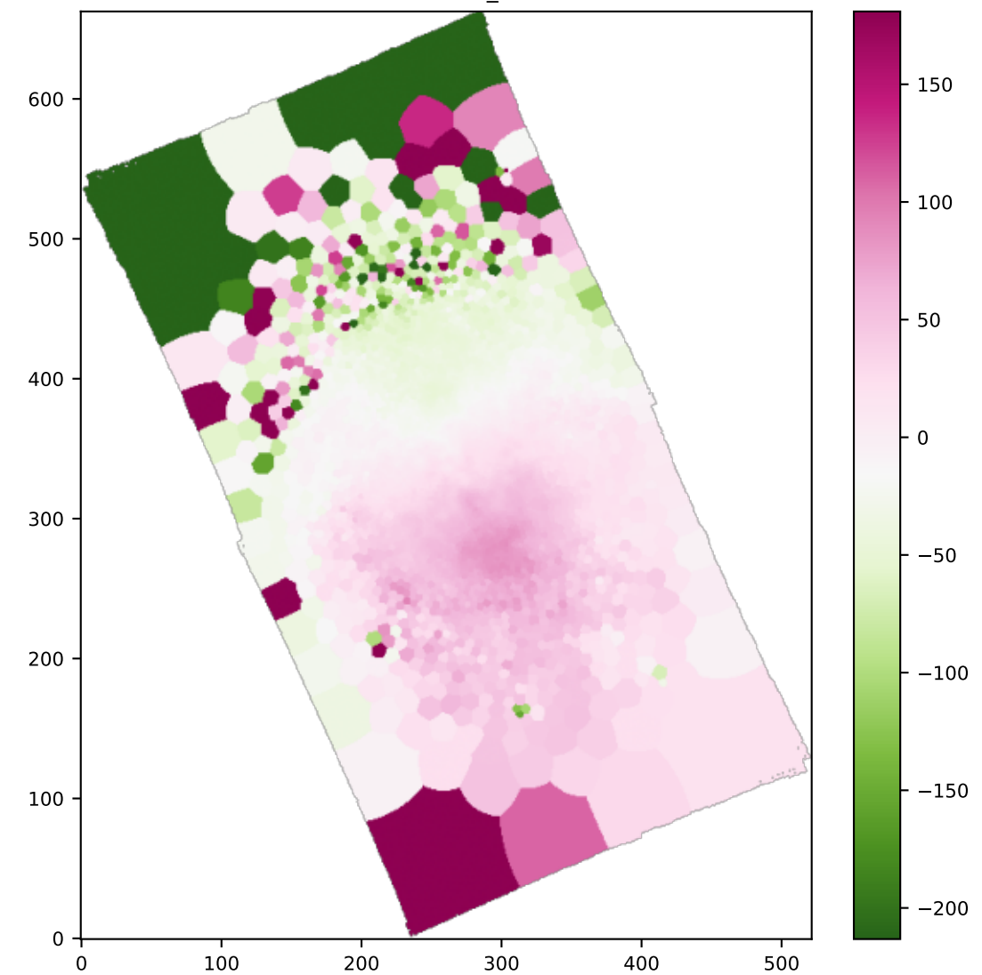
BIN NII6583_VEL
