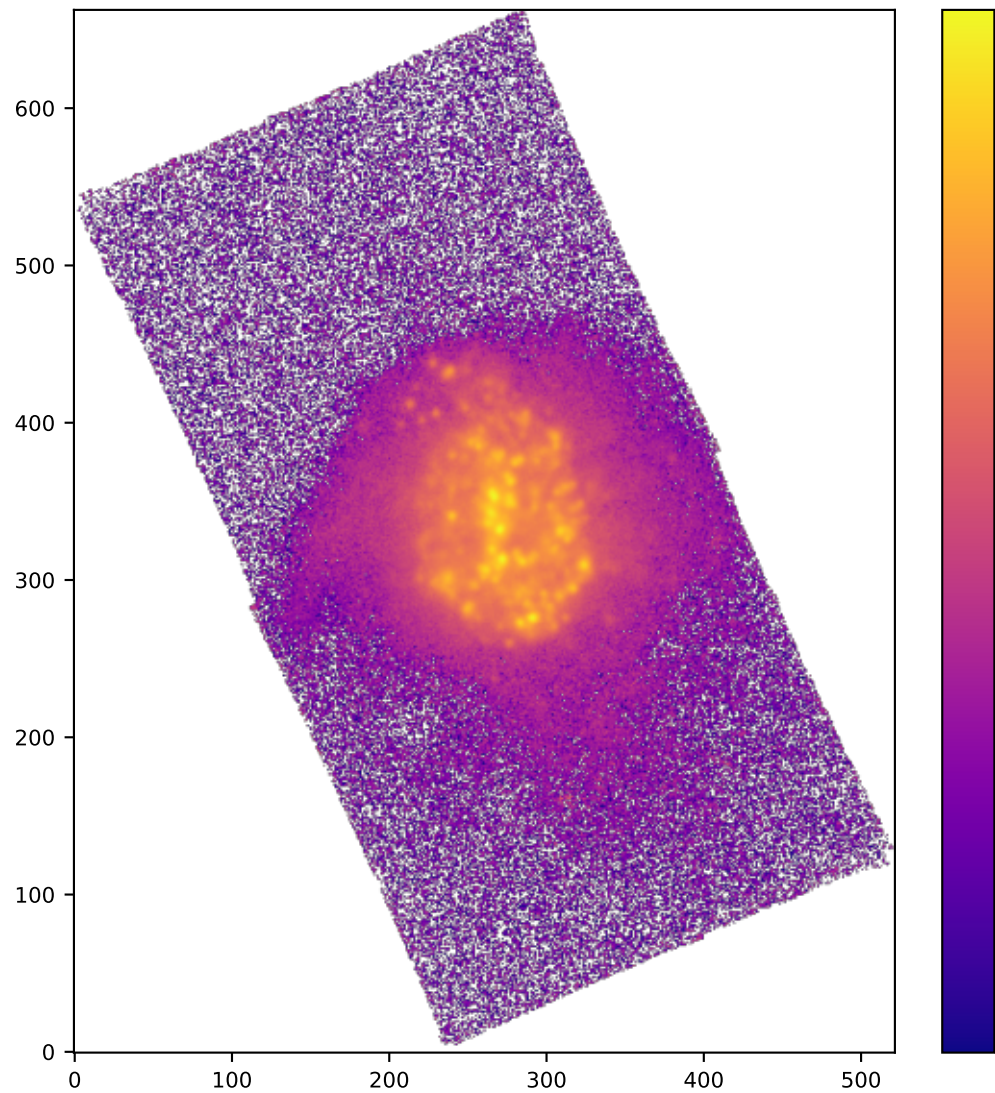
SPAXELS NII6583_SIGMA
