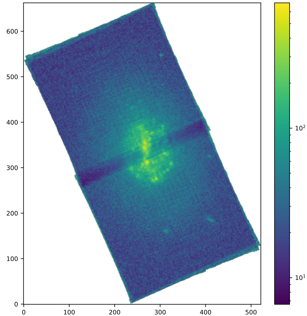
SPAXELS NII6583_SIGMA_ERR
