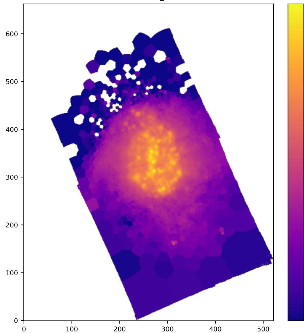
BIN NII6583_SIGMA
