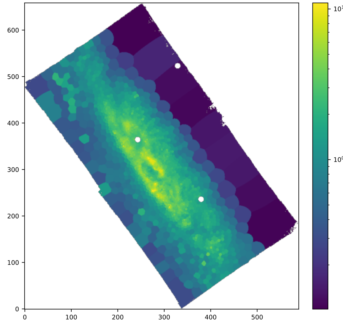
BIN OIII5006_SIGMA_ERR
