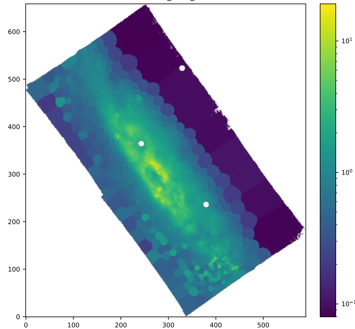
BIN NII6583_SIGMA_ERR
