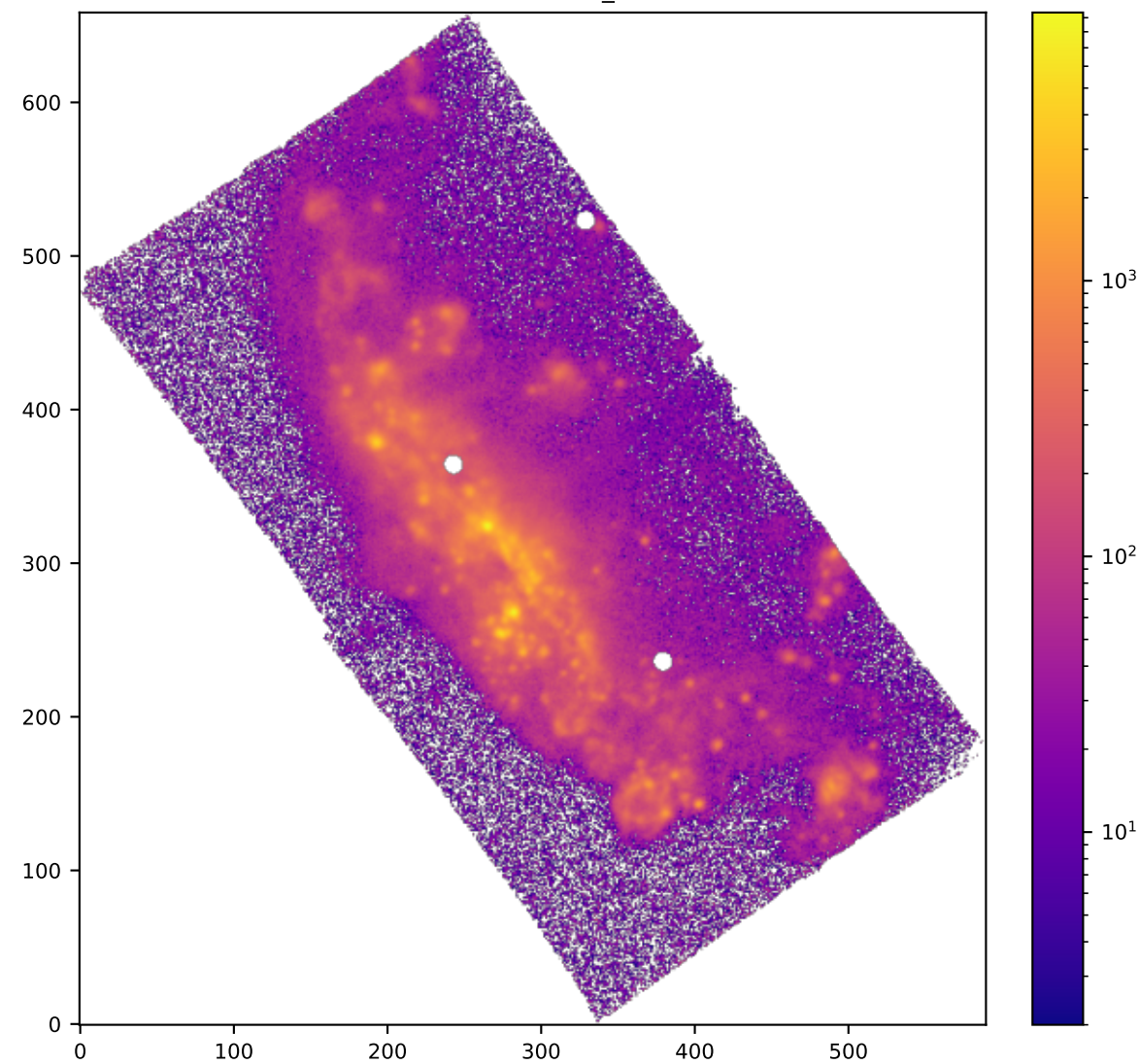
SPAXELS NII6583_SIGMA
