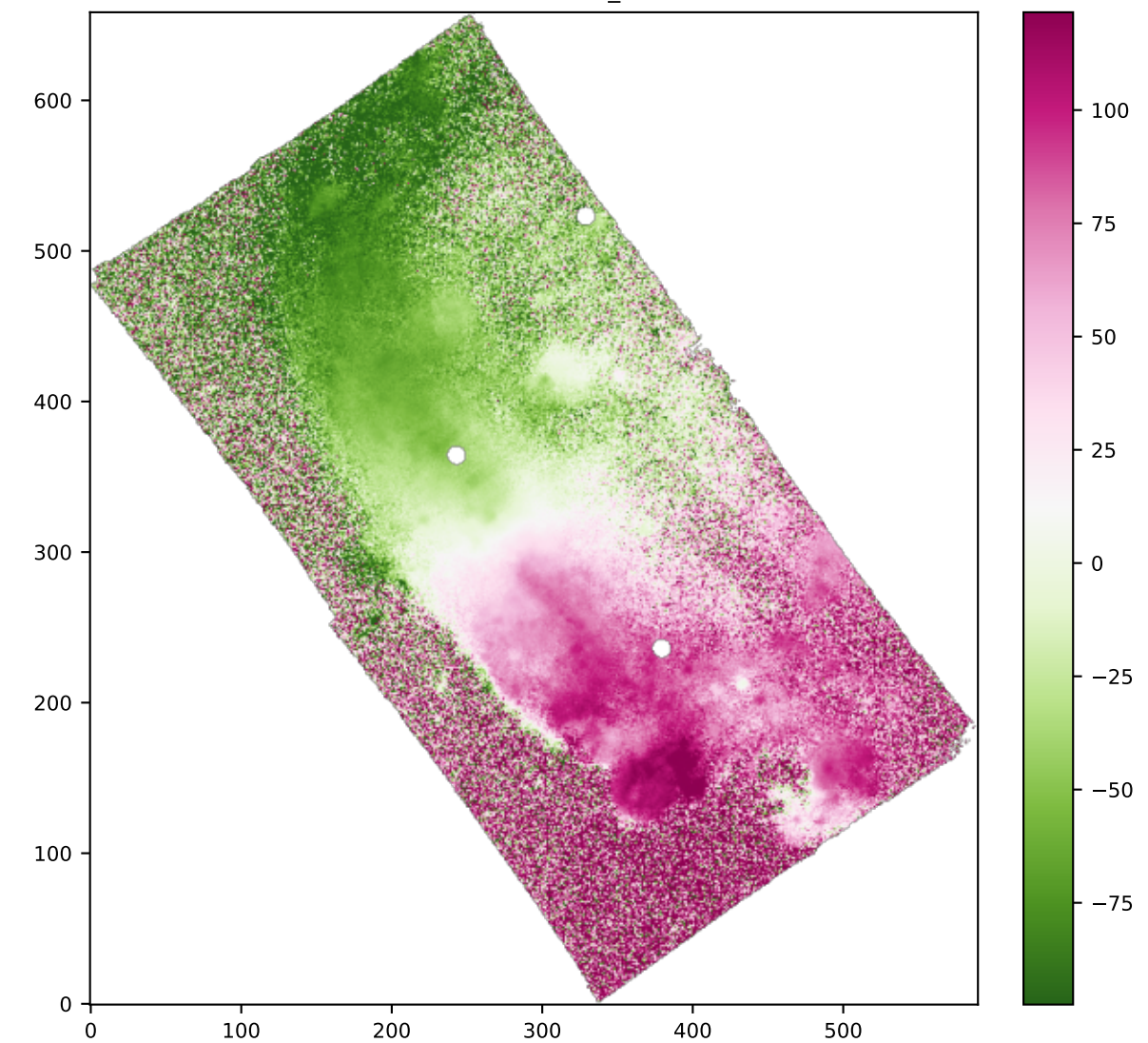
SPAXELS SII6716_VEL
