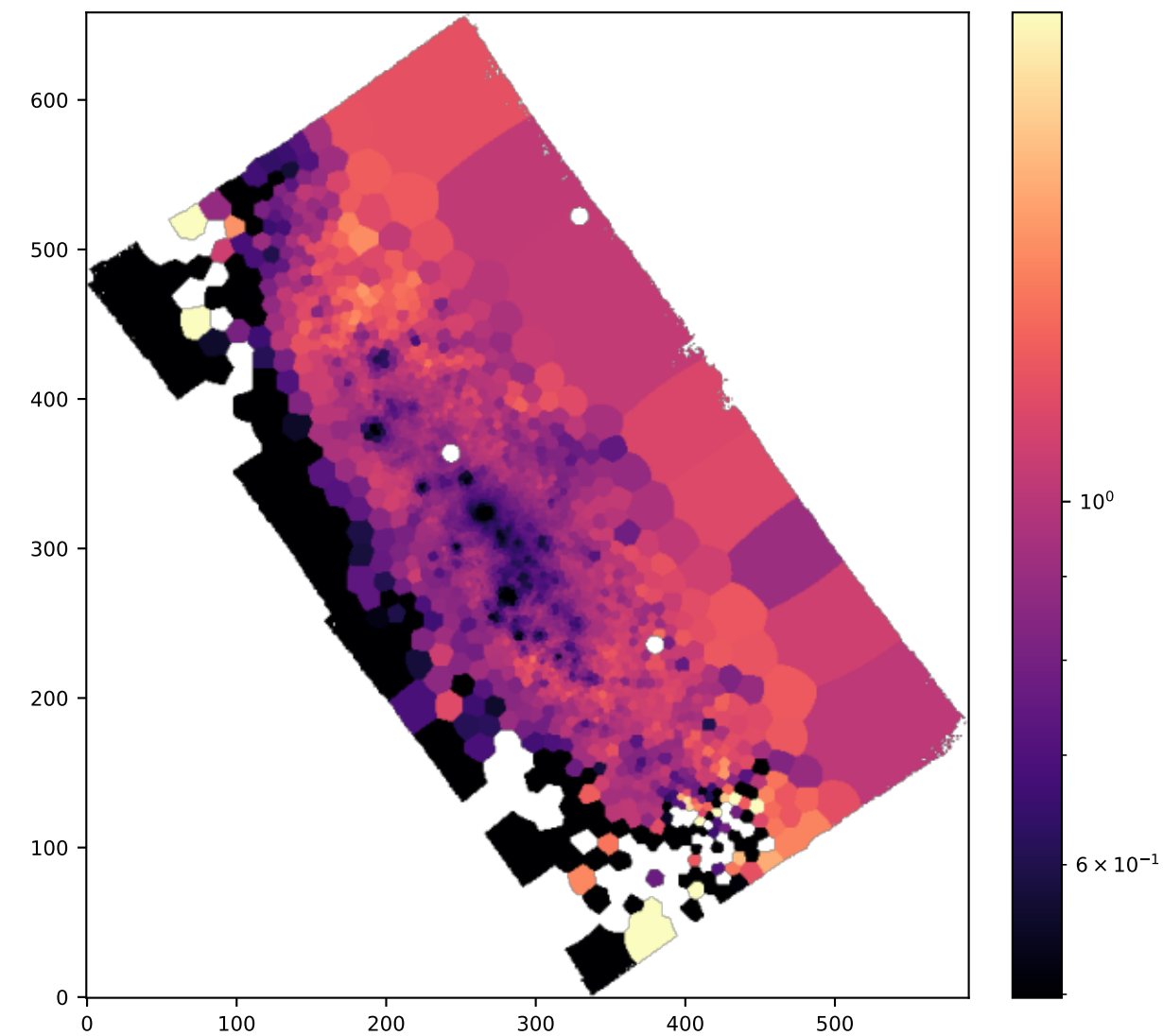
BIN SII/NII
