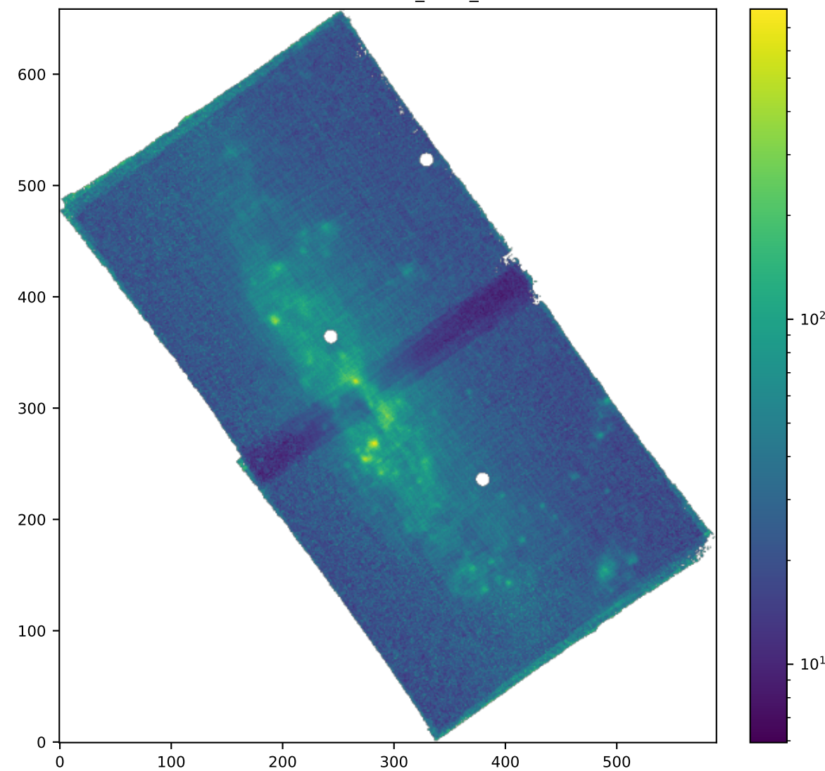
SPAXELS NII6583_SIGMA_ERR
