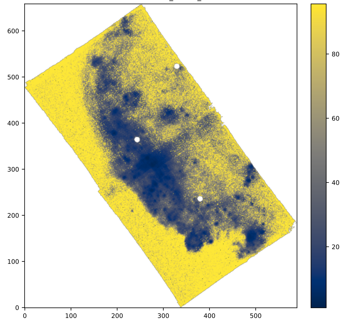
SPAXELS NII6583_SIGMA_ERR
