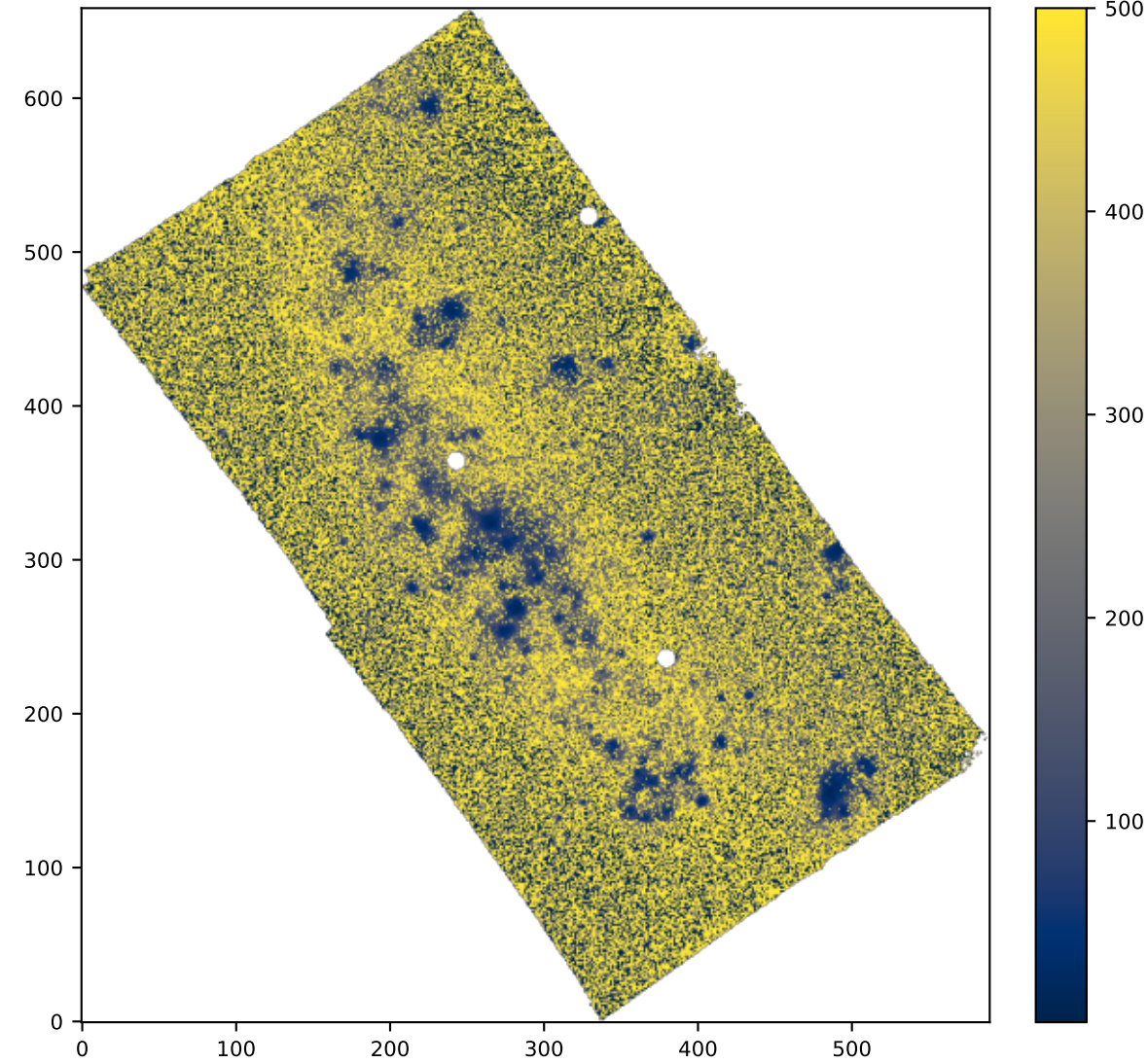
SPAXELS OIII5006_SIGMA_ERR
