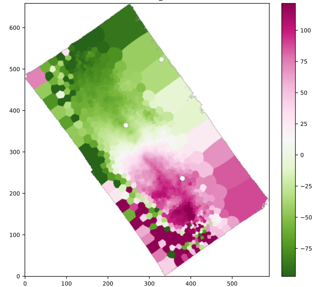
BIN NII6583_VEL
