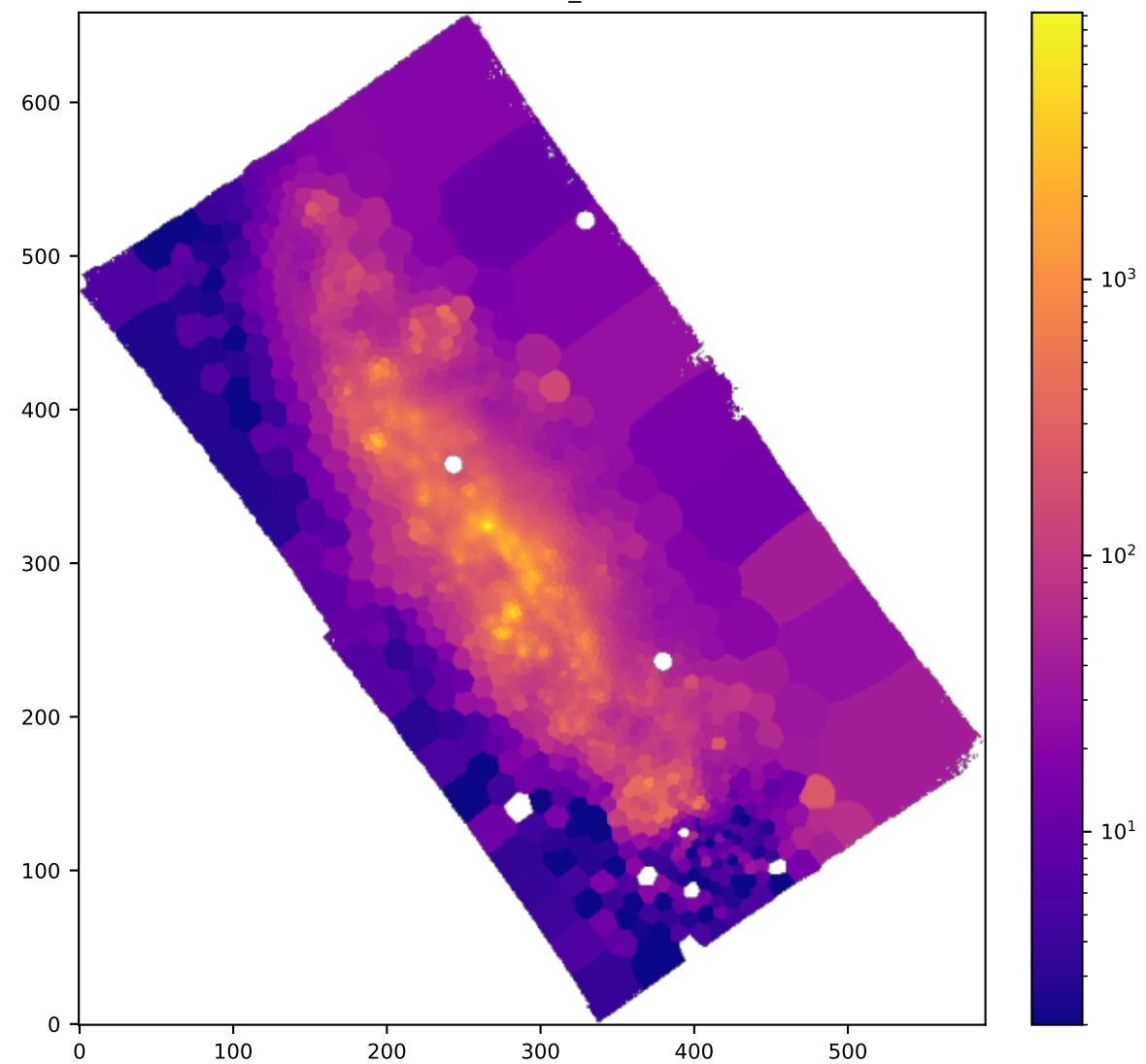
BIN NII6583_SIGMA
