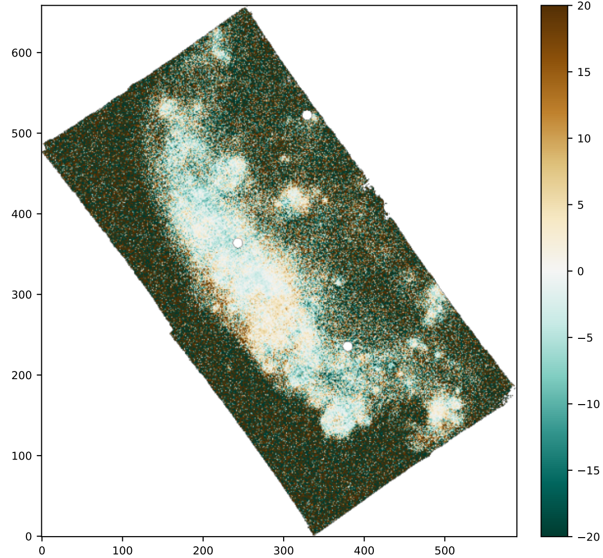
SPAXELS VHa-VNII
