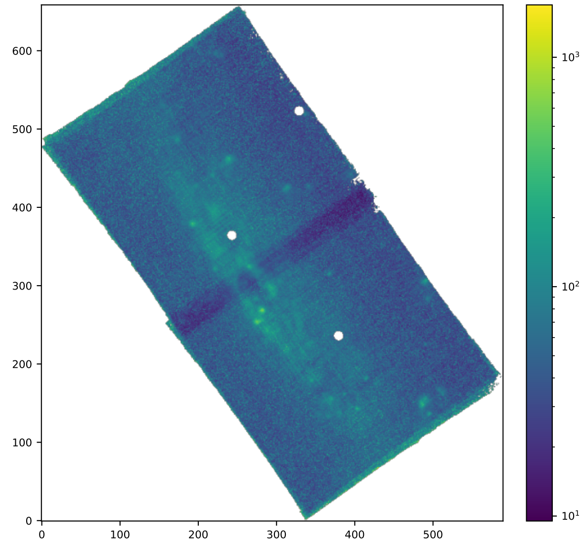
SPAXELS OIII5006_SIGMA_ERR
