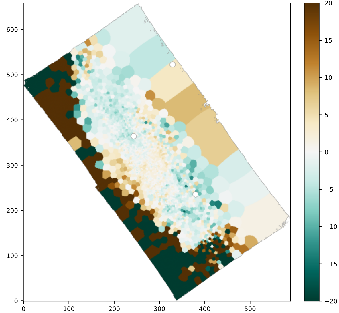
BIN VHa-VNII
