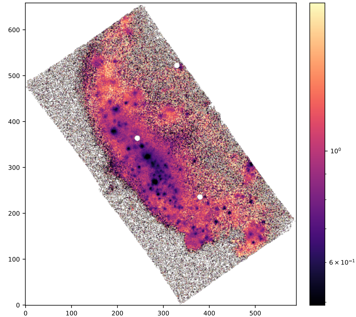
SPAXELS SII/NII
