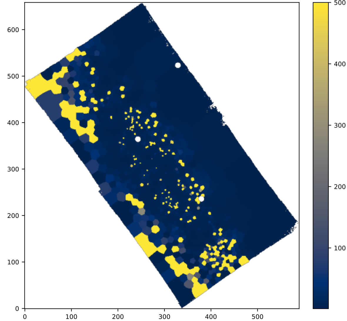
BIN OIII5006_SIGMA_ERR
