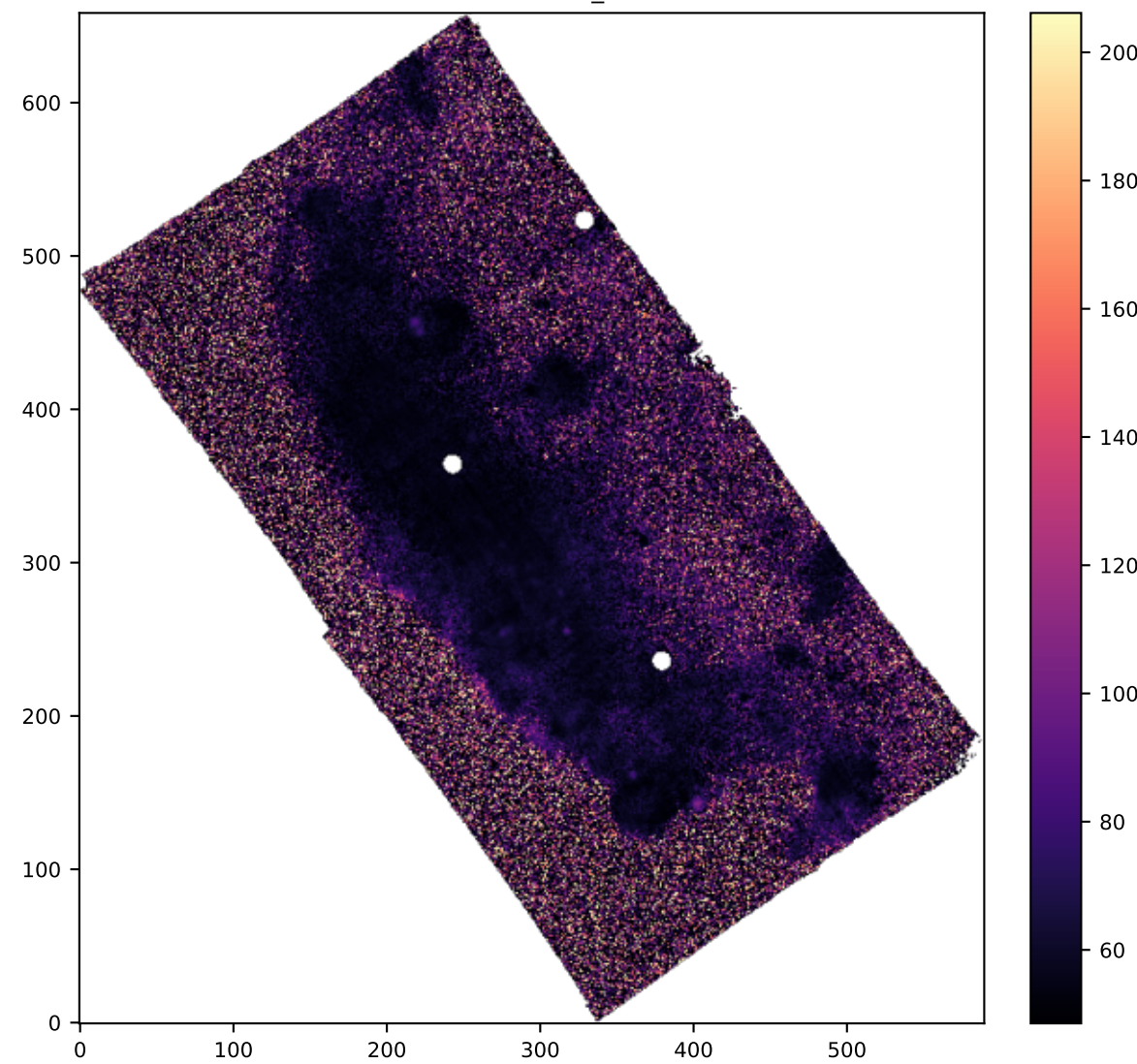
SPAXELS NII6583_SIGMA
