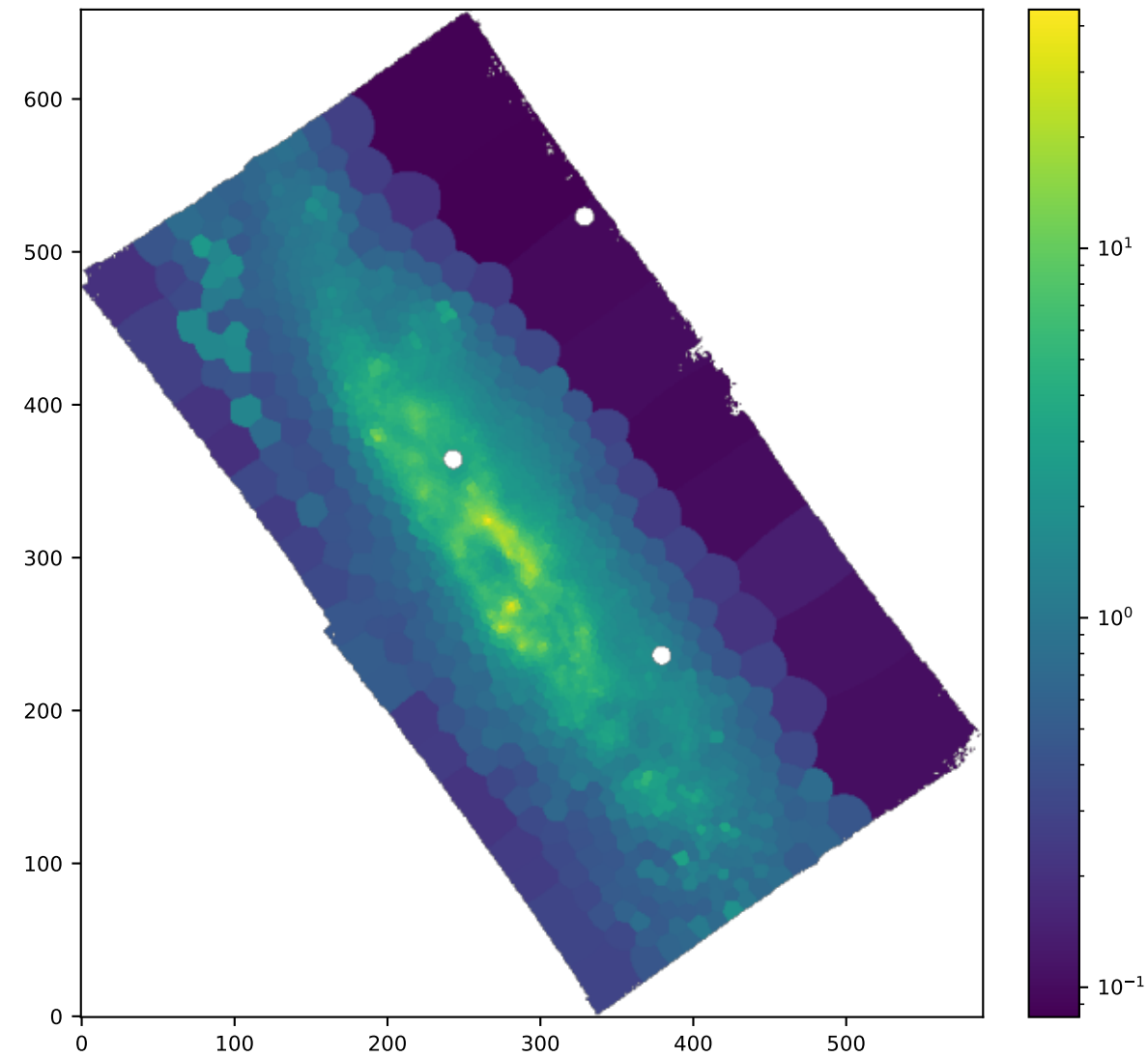
BIN HA6562_SIGMA_ERR
