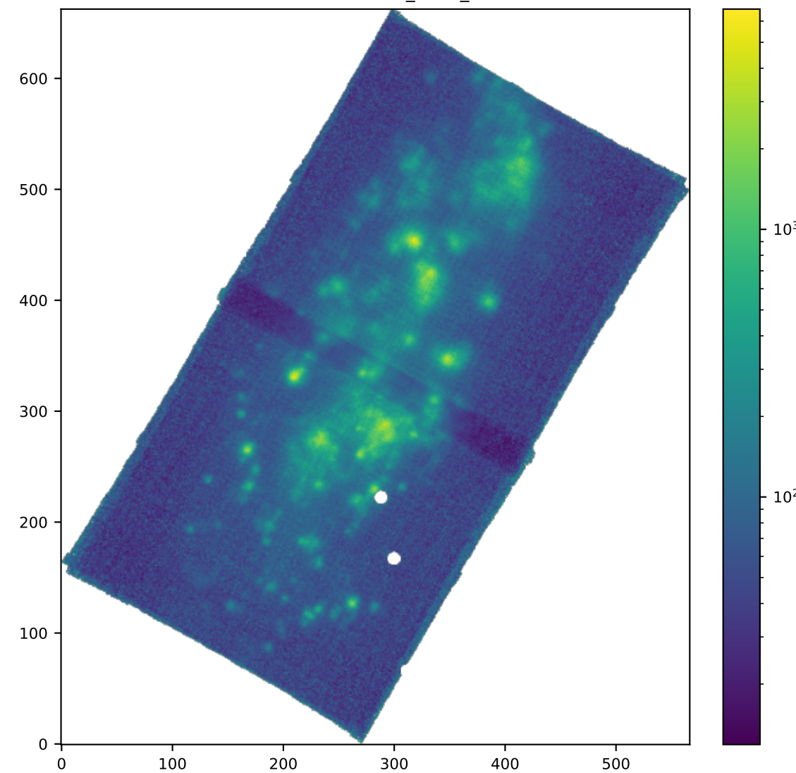
SPAXELS OIII5006_SIGMA_ERR
