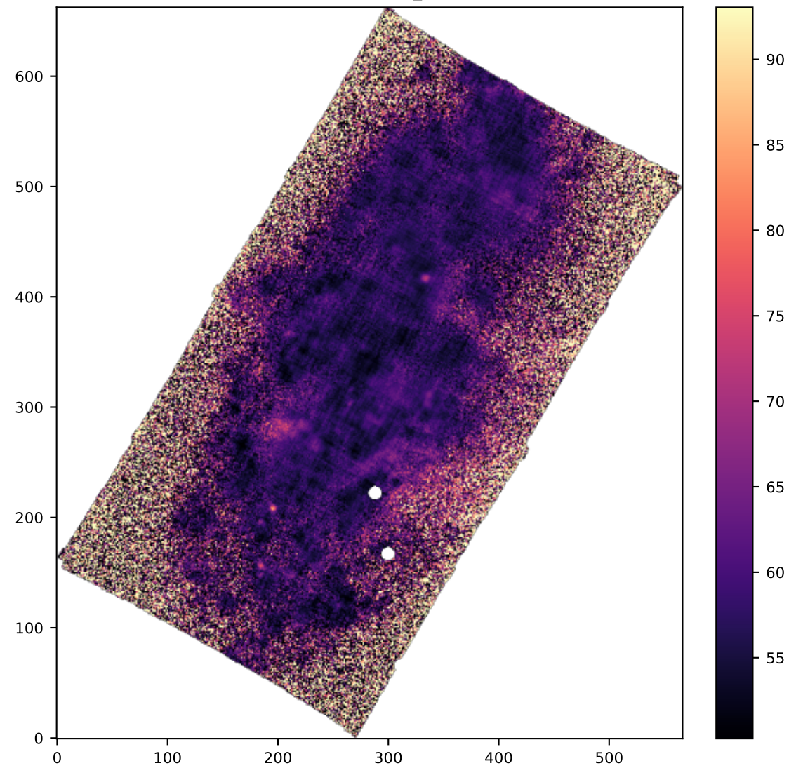
SPAXELS NII6583_SIGMA
