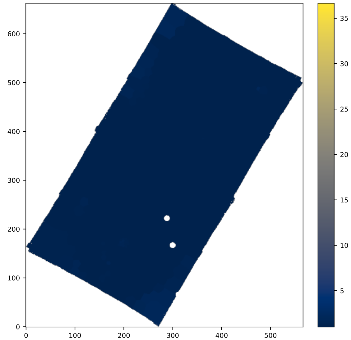
BIN HA6562_SIGMA_ERR
