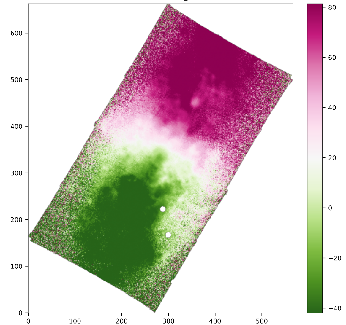
SPAXELS SII6716_VEL
