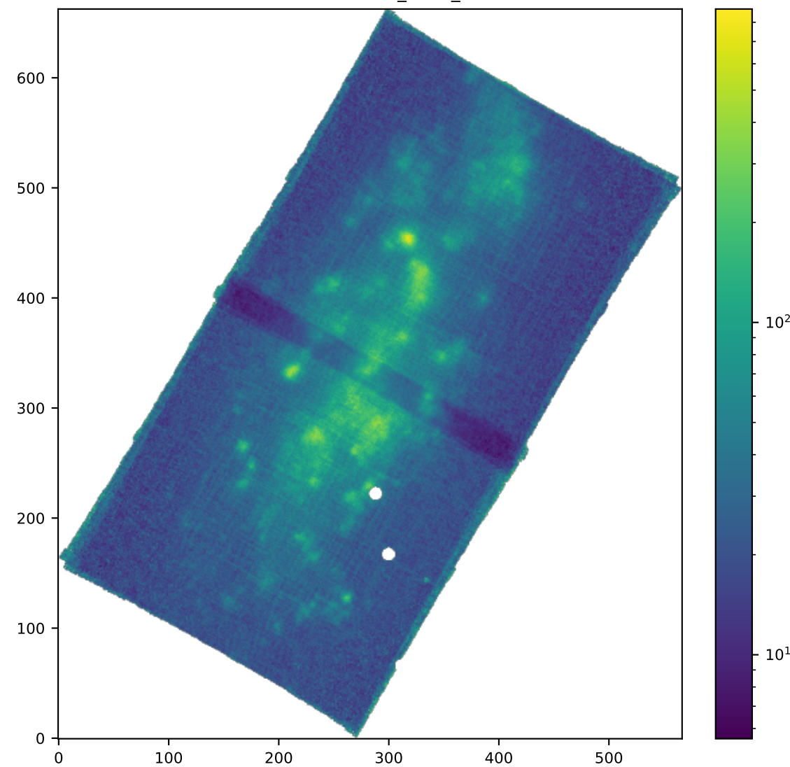
SPAXELS NII6583_SIGMA_ERR
