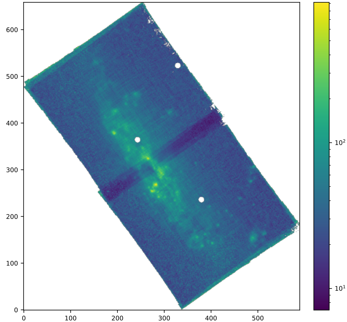
SPAXELS NII6583_SIGMA_ERR
