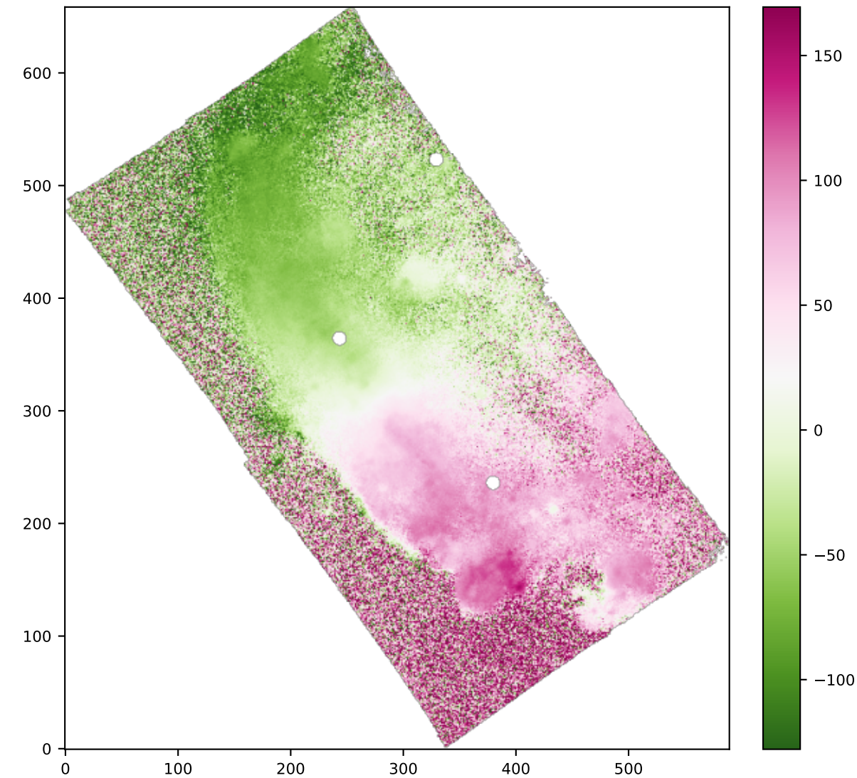
SPAXELS SII6716_VEL
