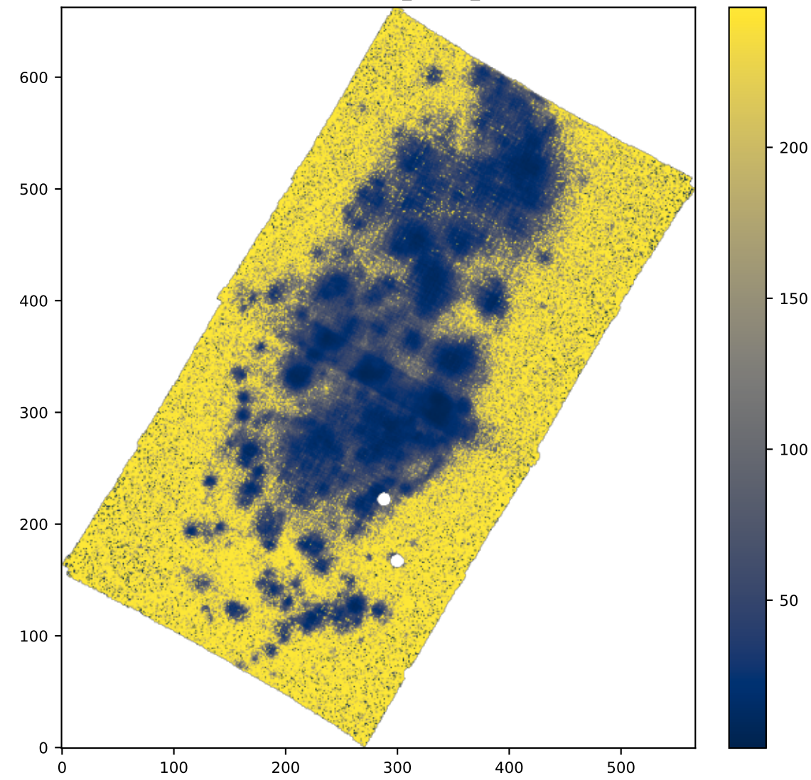
SPAXELS OIII5006_SIGMA_ERR
